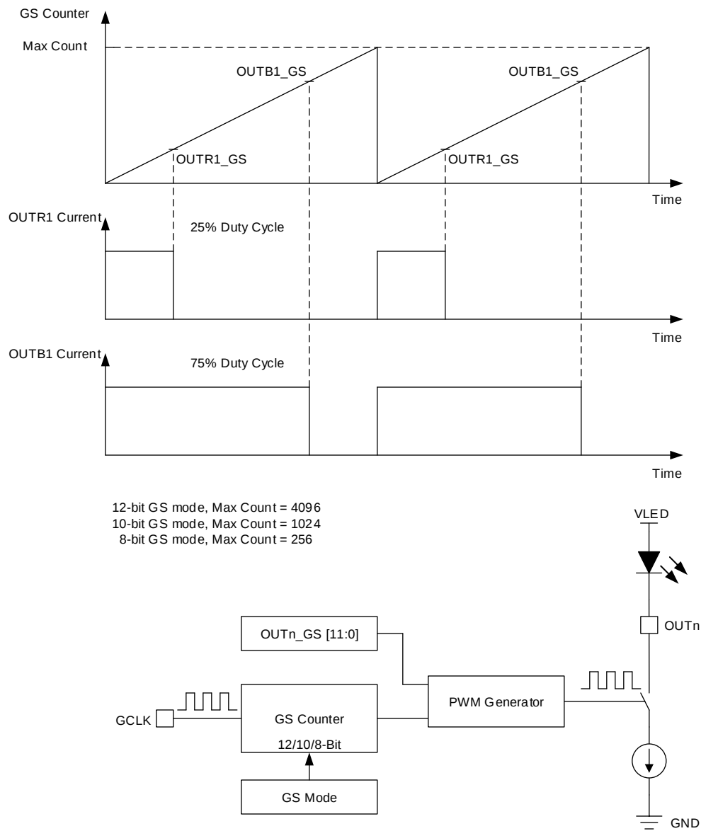
图 22. PWM Generator
