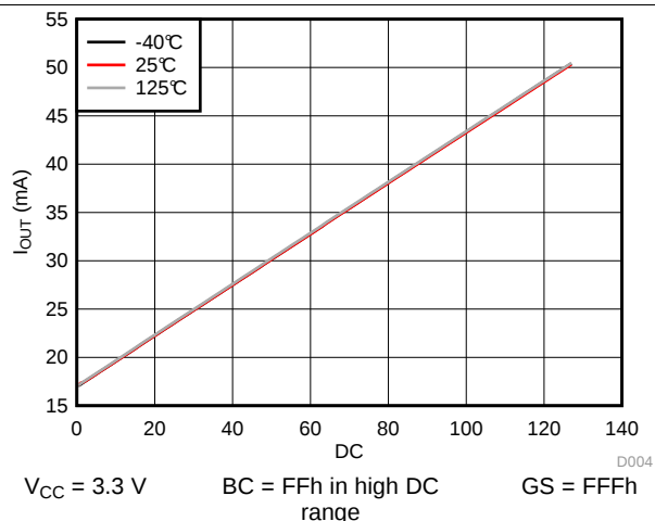
图 18. I_{OUT} vs Dot Correction
