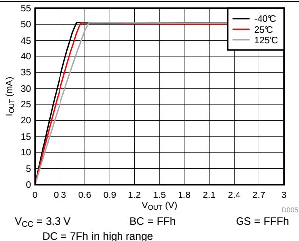
图 16. I_{OUT} vs V_{OUT}
