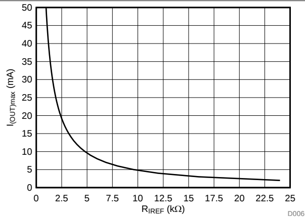
图 15. I_{OUT(max)} vs R_{IREF}
