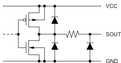
图 6-4. SOUT
