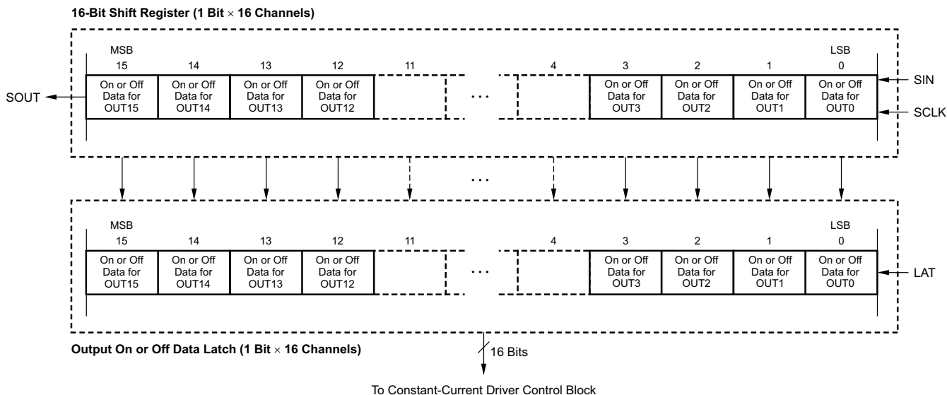
图 8-1. 16 位移位寄存器和输出开关数据锁存器配置
