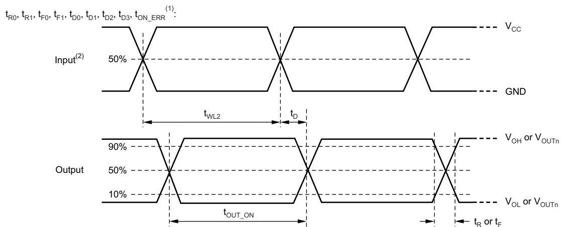
图 5-1. 输入时序图
