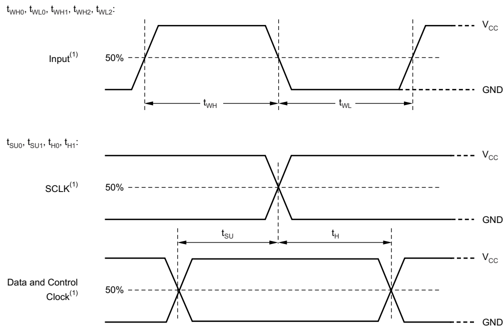
图 5-1. 输入时序图
