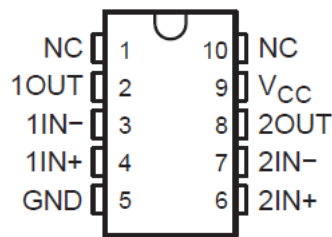
图 4-3. TLC372M U 封装 (顶视图)
