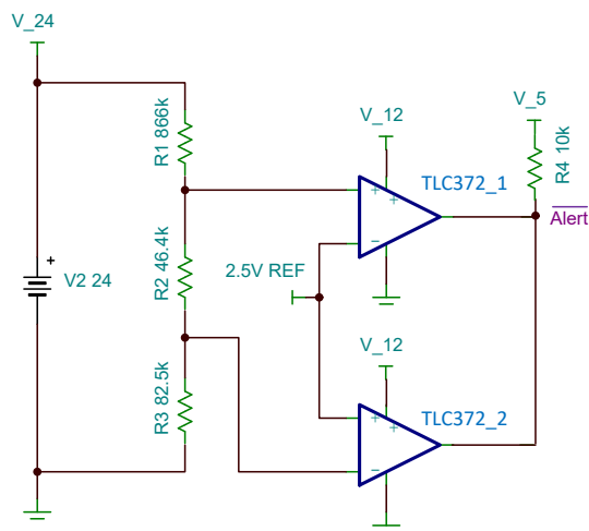
图 8-2. 窗口比较器
