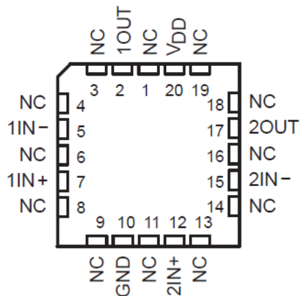
图 4-2. TLC372M FK 封装 (顶视图)
