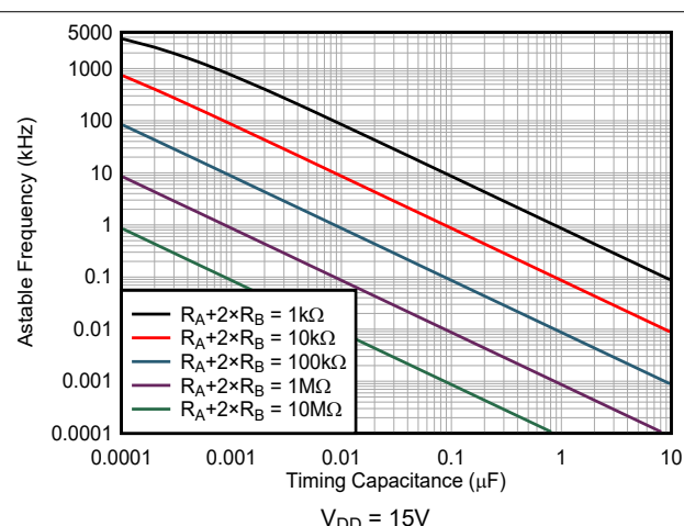
图 6-8. 仿真的非稳态频率
