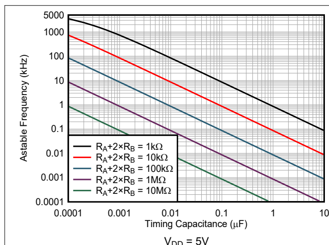
图 6-7. 仿真的非稳态频率
