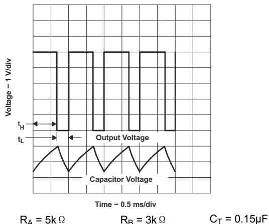
图 6-5. 典型非稳态波形
