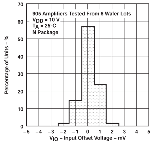
图 5-2. TLC27L4 输入失调电压的分布
