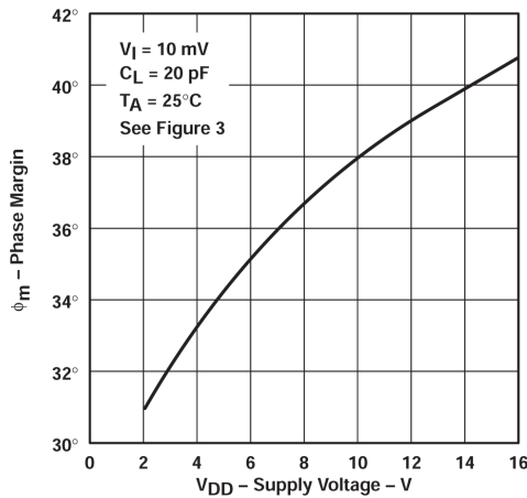
图 5-27. 相位裕度与电源电压间的关系
