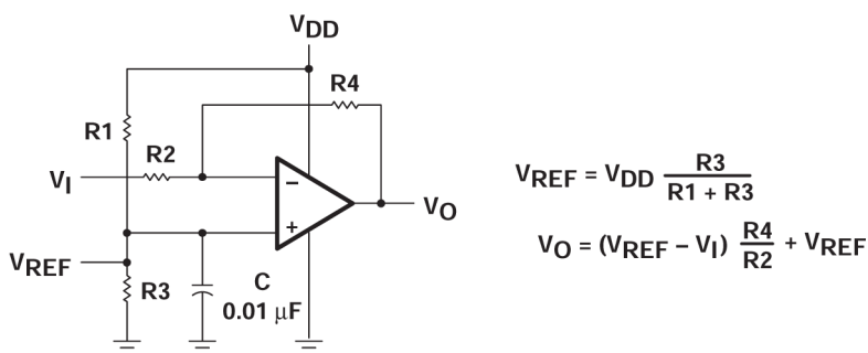
图 7-1. 具有电压基准的反相放大器
