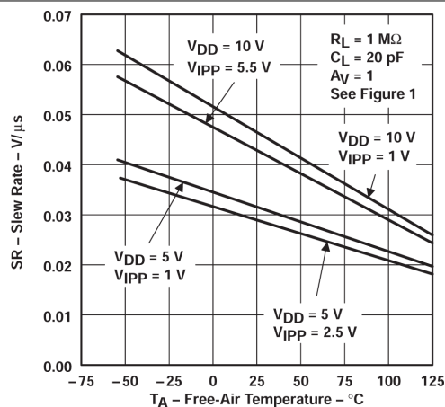
图 5-22. 压摆率与自然通风温度间的关系
