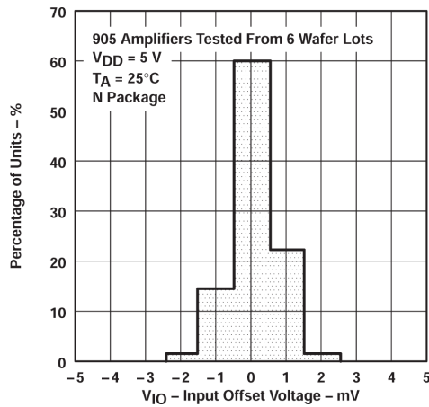
图 5-1. TLC27L4 输入失调电压的分布
