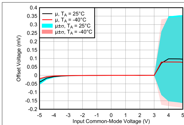
图 7-3. 失调电压与输入共模电压间的关系
