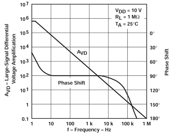
图 5-26. 大信号差分电压放大和相移与频率间的关系
