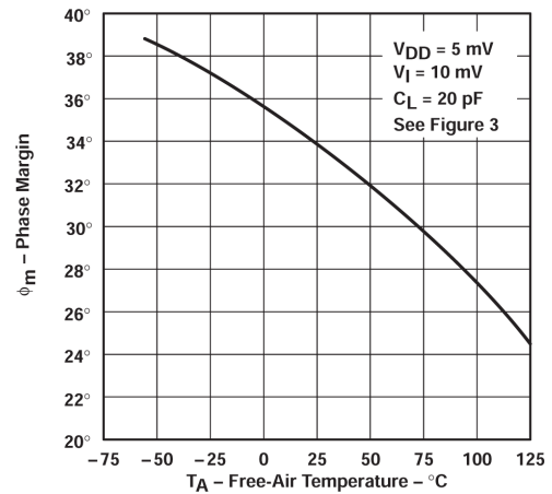
图 5-28. 相位裕度与自然通风温度间的关系
