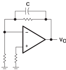
图 7-6. 对输入电容进行补偿
