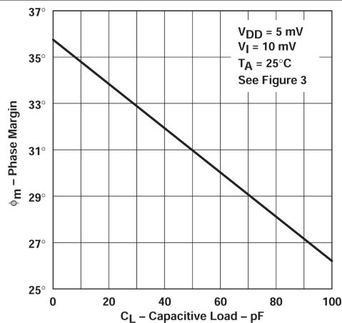
图 5-29. 相位裕度与容性负载间的关系
