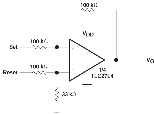
图 7-10. 设置/复位触发器, V_{DD} = 5V 至 16V
