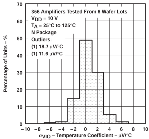
图 5-4. TLC27L4 和 TLC27L9 输入失调电压温度系数的分布
