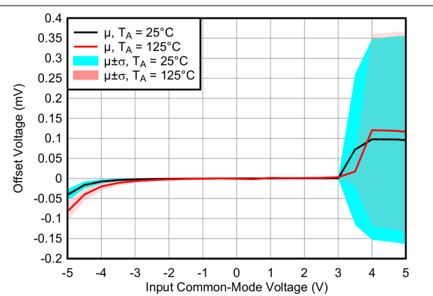
图 7-4. 失调电压与输入共模电压间的关系
