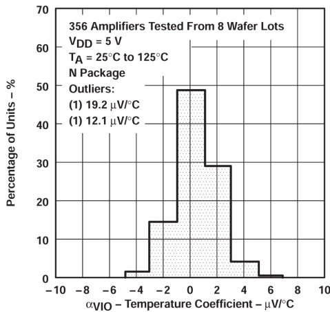
图 5-3. TLC27L4 和 TLC27L9 输入失调电压温度系数的分布
