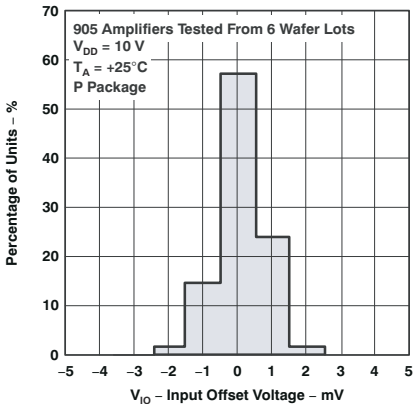
图 5-2. TLC27L1 输入 偏移电压的分布
