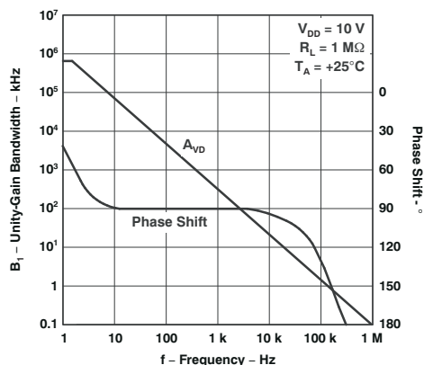
图 5-26. 大信号差动电压 放大和相移 与频率间的关系
