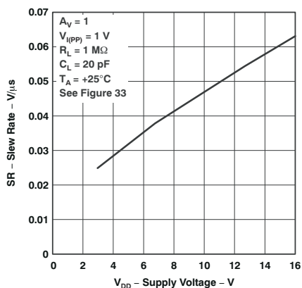
图 5-21. 转换率 与 电源电压间的关系
