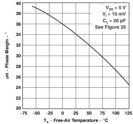
图 5-28. 相位裕度 与 自然通风温度间的关系
