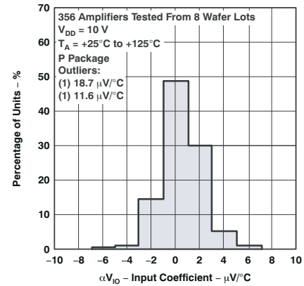
图 5-4. TLC27L1 输入 偏移电压 温度系数的分布
