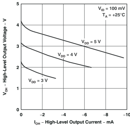
图 5-5. 高电平输出电压 与 高电平输出电流间的关系
