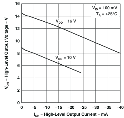
图 5-6. 高电平输出电压 与 高电平输出电流间的关系
