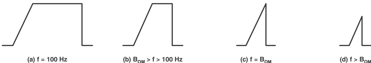
图 6-5. 全功率响应输出信号
