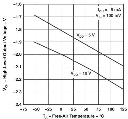
图 5-8. 高电平输出电压 与 自然通风温度间的关系
