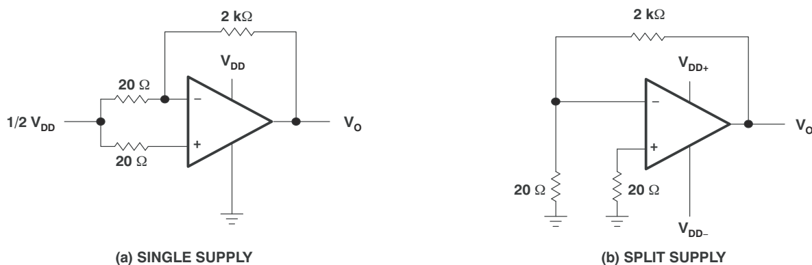
图 6-2. 噪声测试电路
