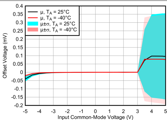
图 7-3. 偏移电压与输入共模电压间的关系
