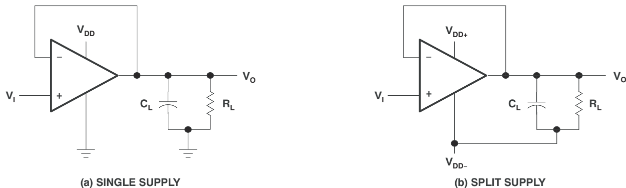
图 6-1. 单位增益放大器
