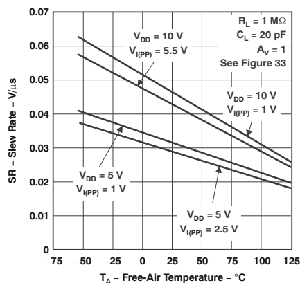
图 5-22. 转换率 与 自然通风温度间的关系
