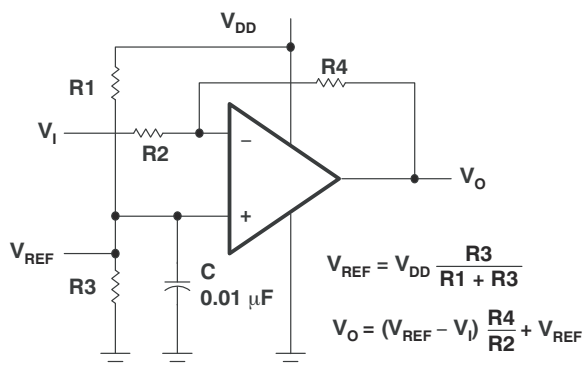
图 7-1. 具有电压基准的反相放大器
