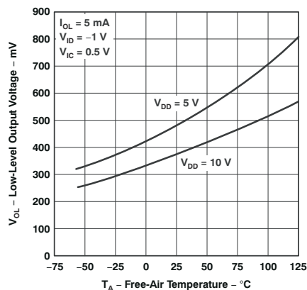
图 5-12. 低电平输出电压 与 自然通风温度间的关系
