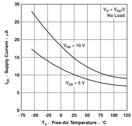
图 5-20. 电源电流 与 自然通风温度间的关系
