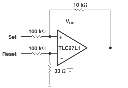
图 7-14. 设置/复位触发器
