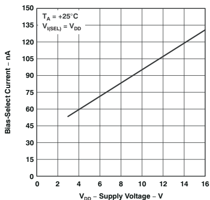
图 5-23. 偏置选择电流 与 电源电压间的关系
