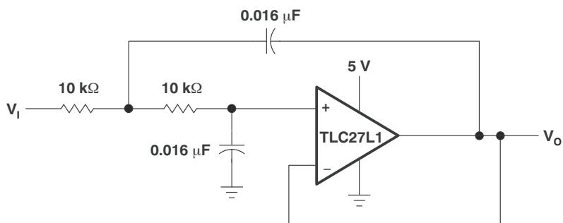
图 7-15. 两极点低通巴特沃斯滤波器
