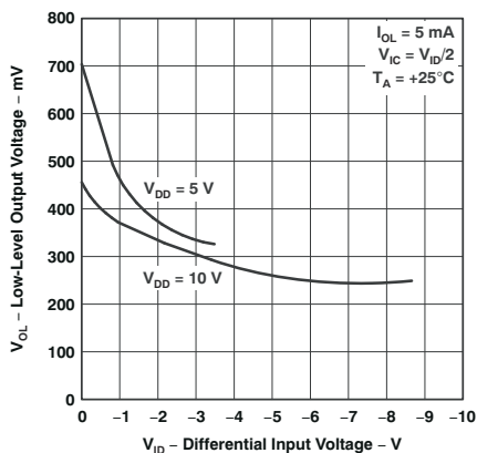
图 5-11. 低电平输出电压 与 差动输入电压间的关系
