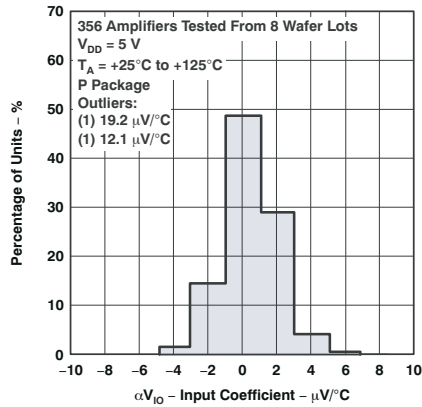
图 5-3. TLC27L1 输入 偏移电压 温度系数的分布
