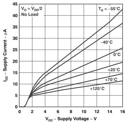
图 5-19. 电源电流 与 电源电压间的关系
