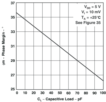
图 5-29. 相位裕度 与 电容负载间的关系
