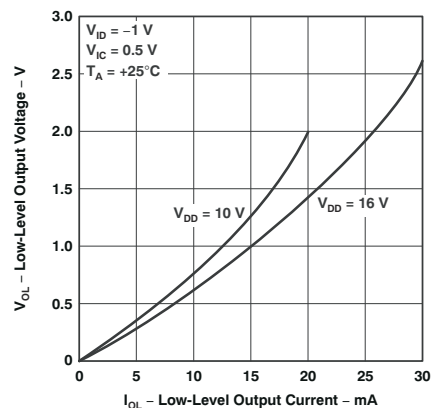
图 5-14. 低电平输出电压 与 低电平输出电流间的关系
