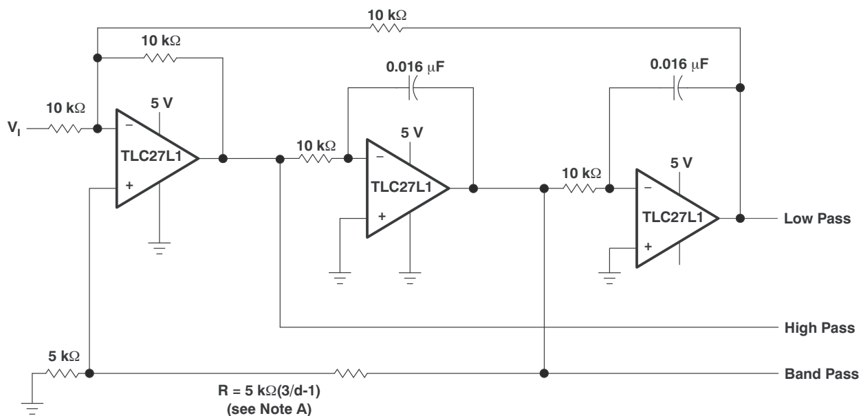
图 7-10. 状态变量滤波器
