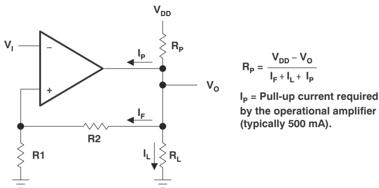
图 7-9. 使用电阻式上拉电阻器来提高 V_{OH}
