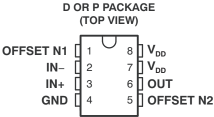
图 4-1. D 封装 ( 8 引脚 SOIC ) 或 P 封装 ( 8 引脚 PDIP ) ( 俯视图顶视图 )
