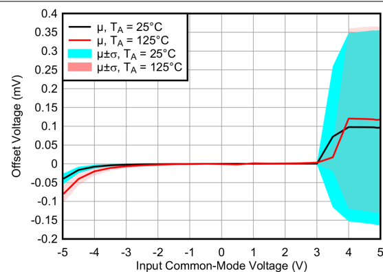
图 7-4. 偏移电压与输入共模电压间的关系
