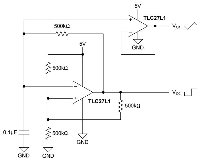
图 7-12. 多谐振荡器
