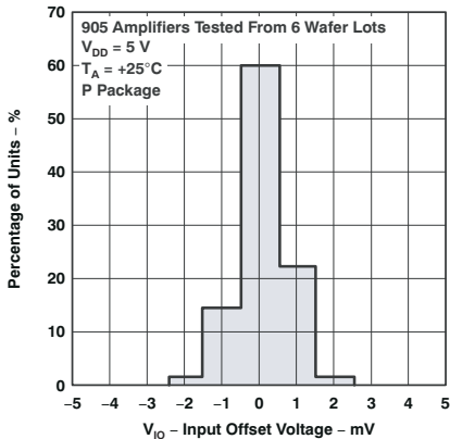
图 5-1. TLC27L1 输入 偏移电压的分布
