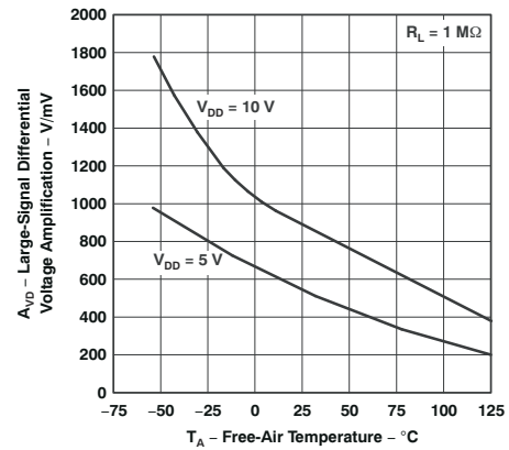
图 5-16. 大信号 差动电压放大 与自然通风温度间的关系
