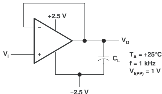
图 7-7. 输出特性测试电路
