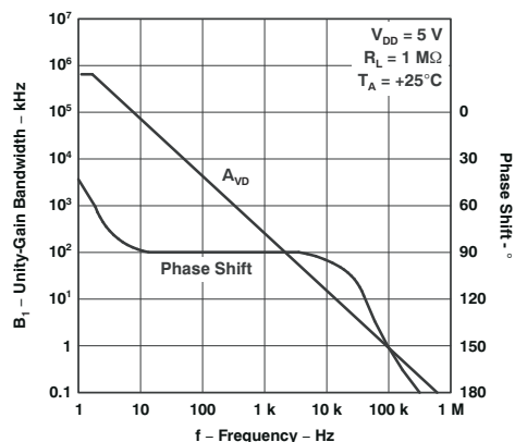
图 5-25. 大信号差动电压 放大和相移 与频率间的关系
