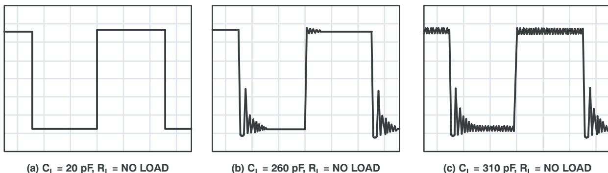
图 7-8. 低偏置模式下电容负载的影响
