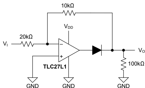
图 7-13. 全波整流器
