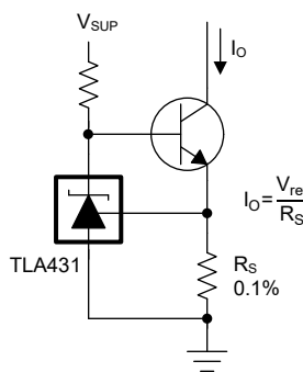
图 9-10. 精密恒定电流吸收器
