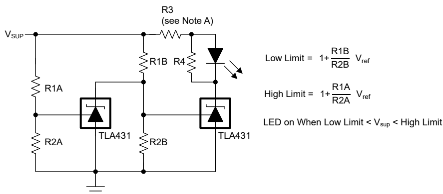
图 9-8. 电压监控器
