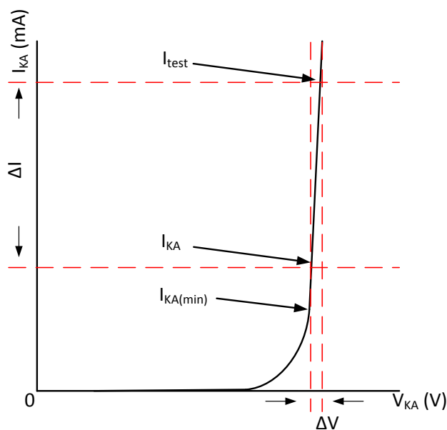
图 7-4. 动态阻抗
