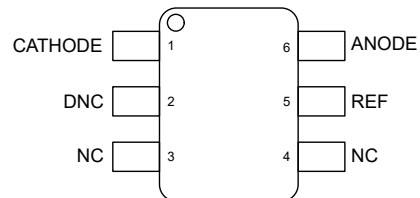
图 5-3. DRL 封装、 6 引脚 SOT-563、TLA431 (顶视图) 产品预览
