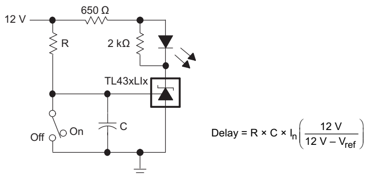
图 35. 延迟计时器
