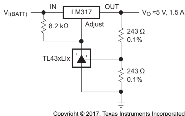
图 31. 精密 5V 1.5A 稳压器
