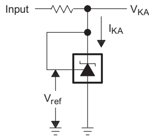
简化原理图
