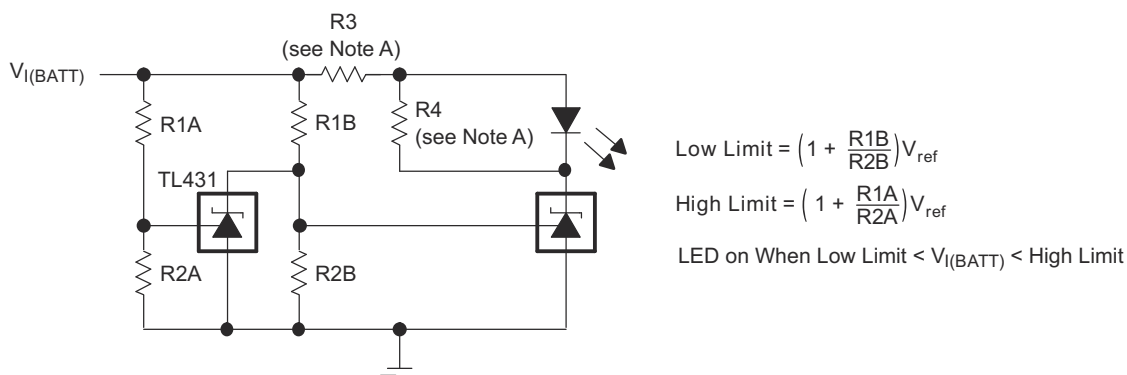
图 9-12. 电压监控器
