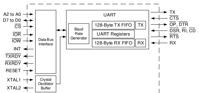
方框图
