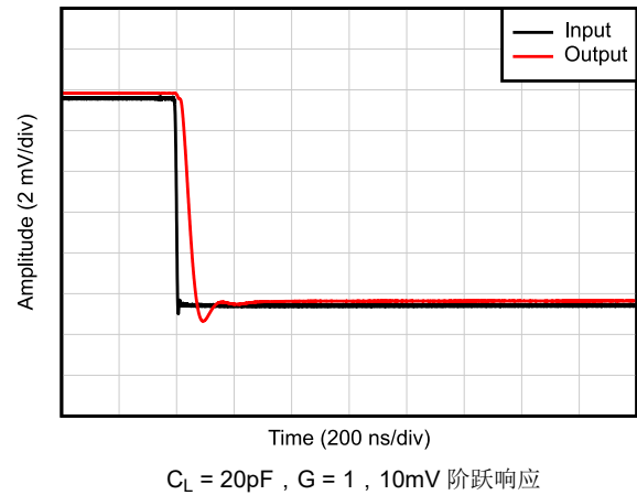
图 5-30. 小信号阶跃响应，下降
