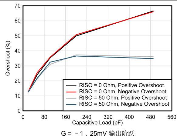
图 5-23. 小信号过冲与容性负载间的关系
