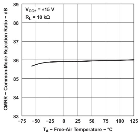
图 6-50. 共模抑制比与自然通风温度间的关系
