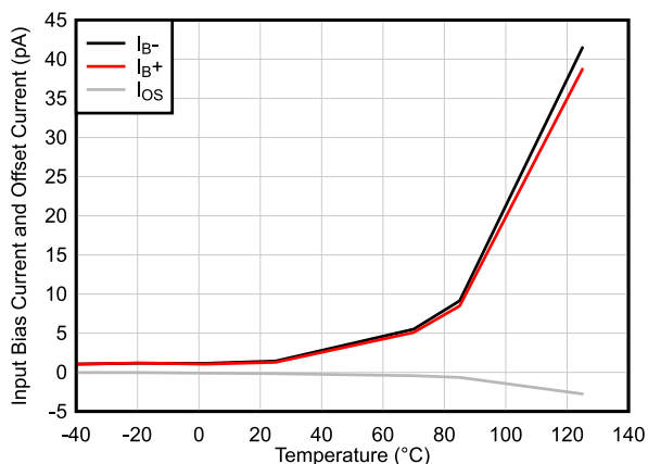
图 6-11. 输入偏置电流与温度间的关系
