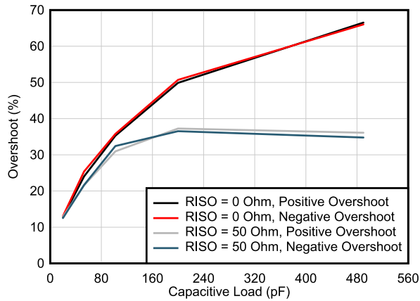
图 6-25. 小信号过冲与容性负载间的关系
