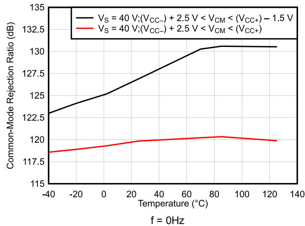
图 6-15. CMRR 与温度间的关系 (dB)
