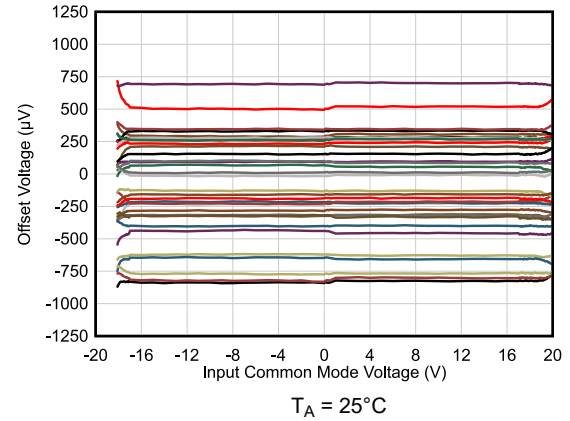
图 6-4. 失调电压与共模电压间的关系
