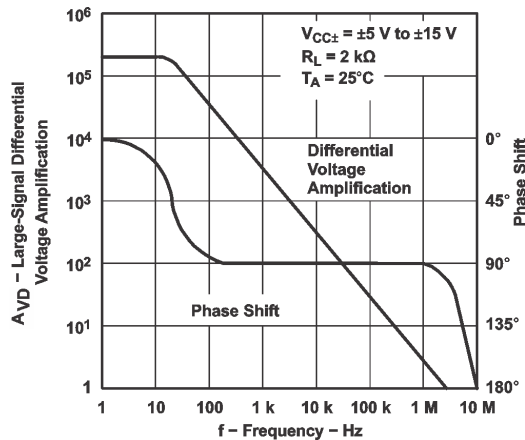
图 6-48. 大信号差分电压放大和相移与频率间的关系
