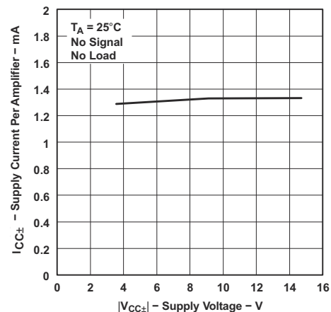
图 6-51. 每个放大器的电源电流与电源电压间的关系
