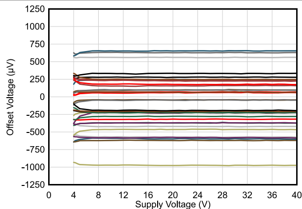
图 6-7. 失调电压与电源间的关系
