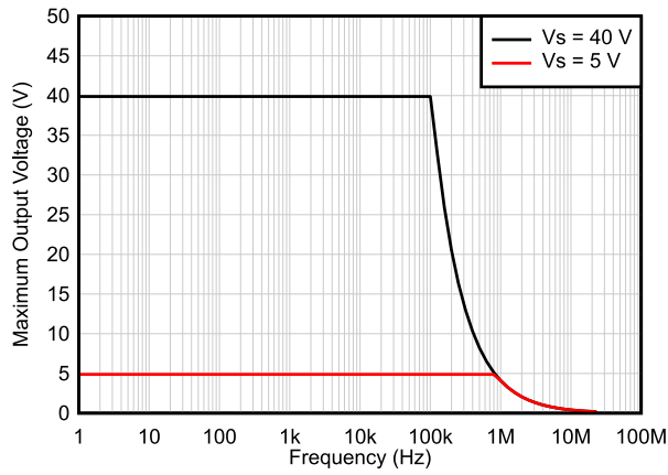
图 6-37. 最大输出电压与频率间的关系
