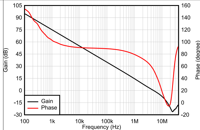
图 6-8. 开环增益和相位与频率间的关系
