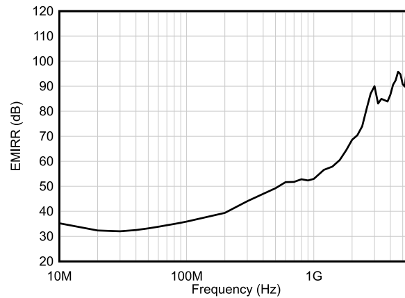
图 6-39. EMIRR (电磁干扰抑制比) 与频率间的关系
