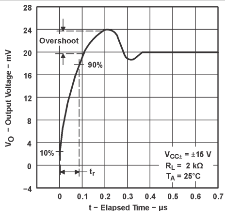
图 6-58. 输出电压与经历时间的关系
