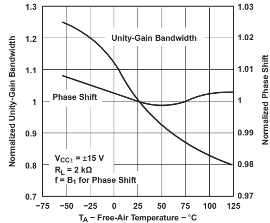
图 6-49. 标称单位增益带宽和相移与自然通风温度间的关系
