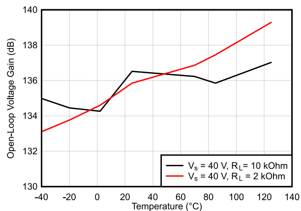
图 6-23. 开环电压增益与温度间的关系 (dB)
