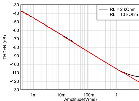
图 6-20. THD+N 与输出幅度间的关系
