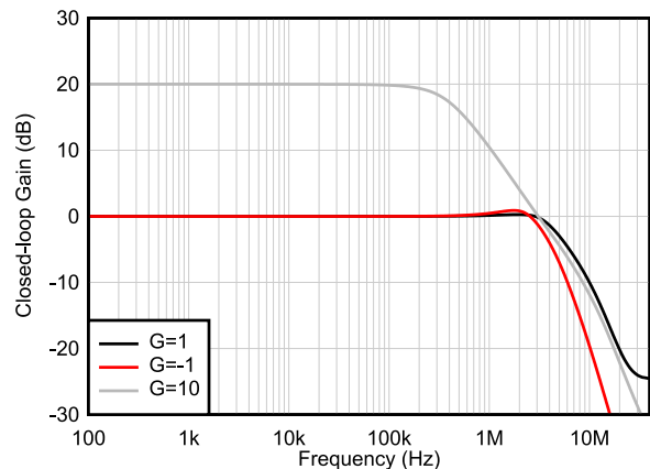
图 6-9. 闭环增益与频率间的关系
