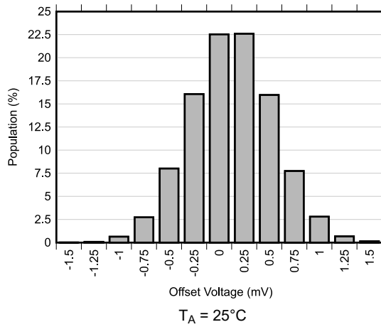
图 6-1. 失调电压产生分布
