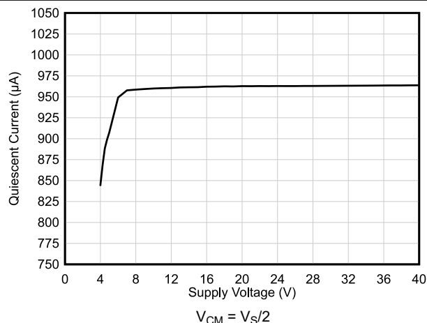
图 6-21. 静态电流与电源电压间的关系
