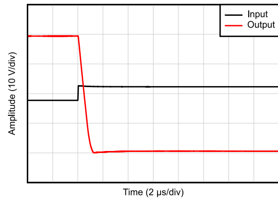
图 6-30. 负过载恢复
