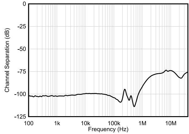
图 6-38. 通道隔离与频率间的关系
