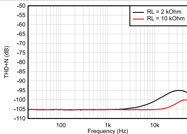
图 6-19. THD+N 比与频率间的关系
