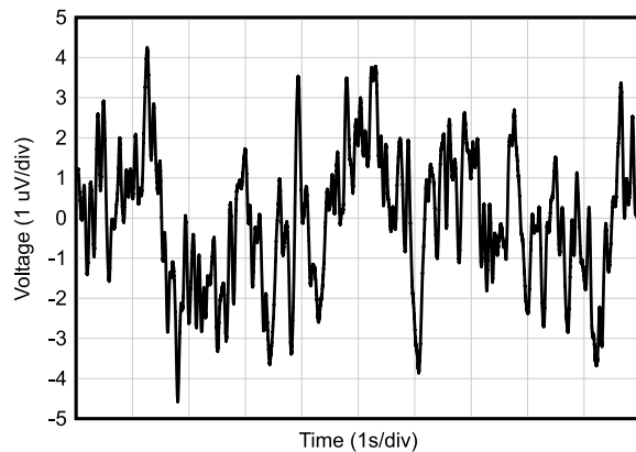
图 6-17. 0.1Hz 至 10Hz 噪声
