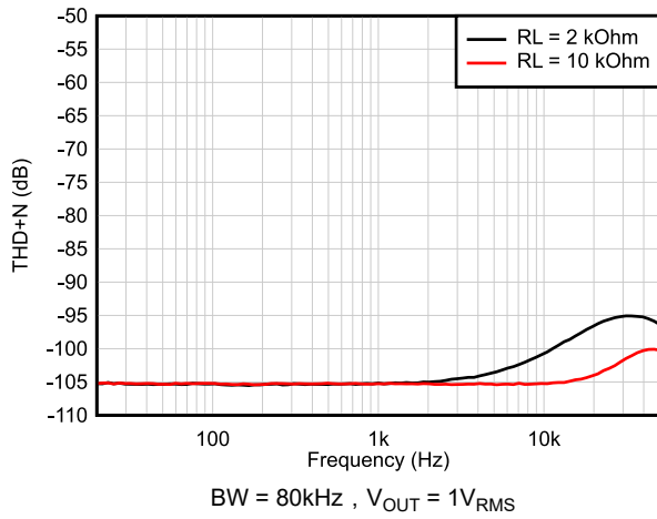
图 6-19. THD+N 比与频率间的关系
