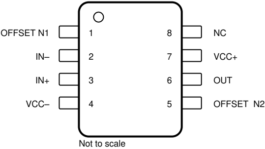
图 4-4. TL071C PS 封装，8 引脚 SO ( 顶视图 )
