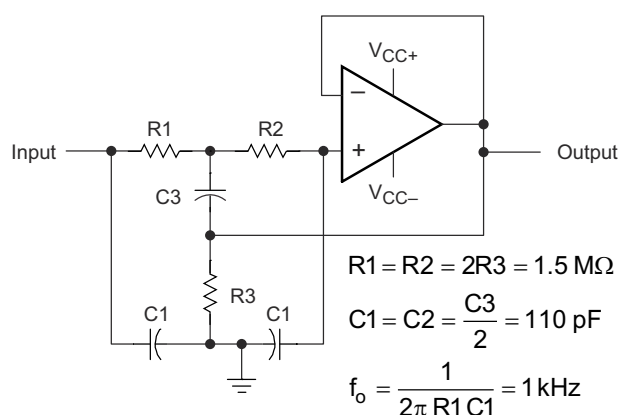
图 9-7. 高 Q 值陷波滤波器
