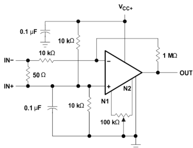
图 9-9. 交流放大器
