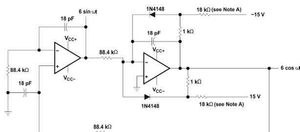
图 9-8. 100kHz 正弦振荡器
