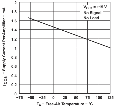
图 6-52. 每个放大器的电源电流与自然通风温度间的关系
