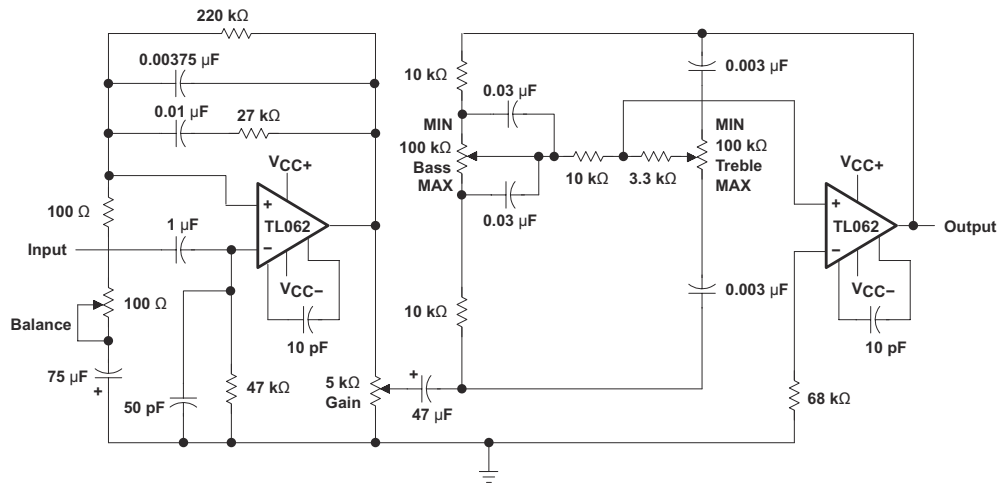
图 9-11. IC Preamplifier
