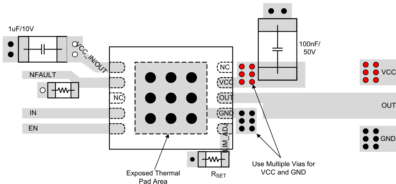
图 11-1. Layout Example
