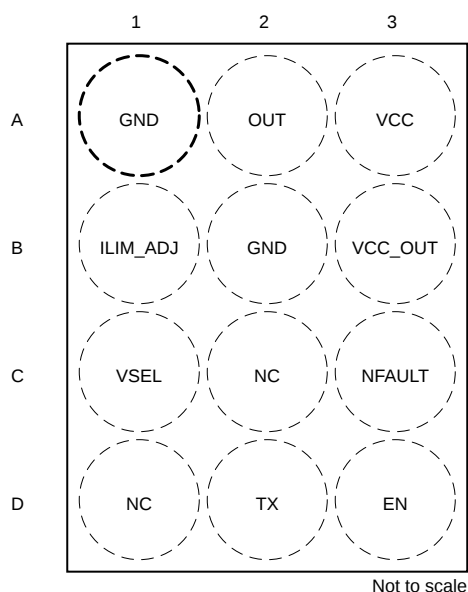
图 5-3. TIO1023L YAH, 12-Pin DSBGA (Top View)
