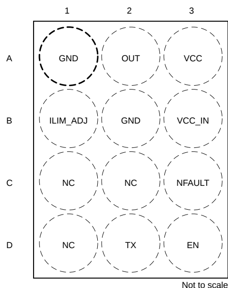
图 5-4. TIO102 YAH, 12-Pin DSBGA (Top View)
