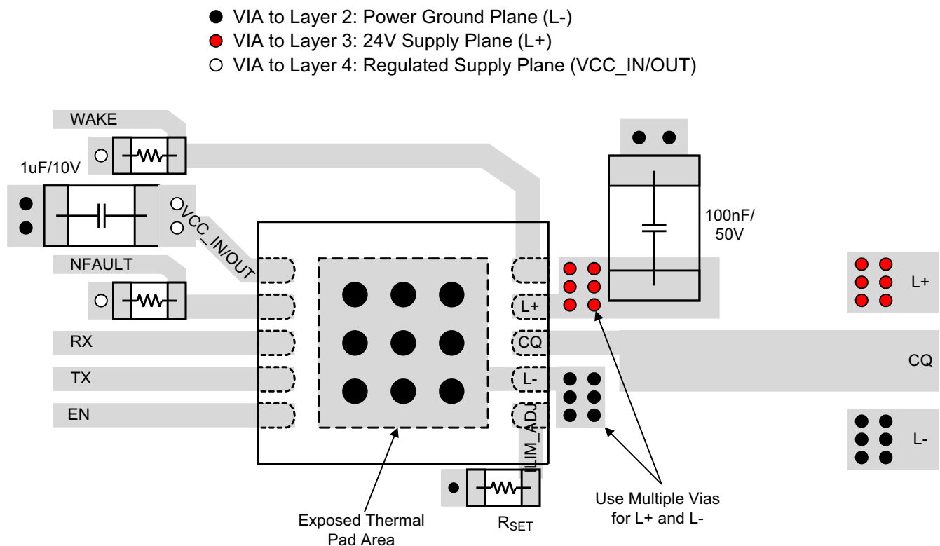
图 9-9. Layout Example
