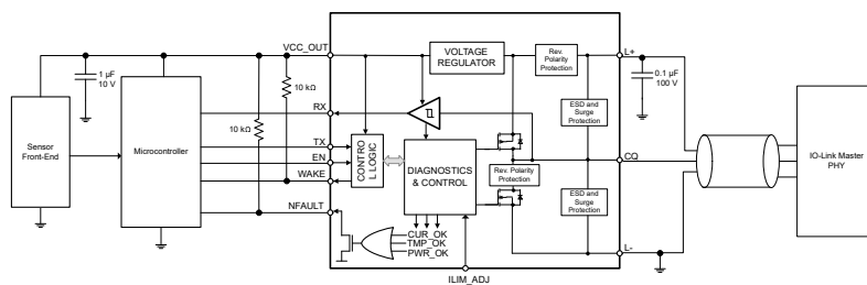
典型应用图
