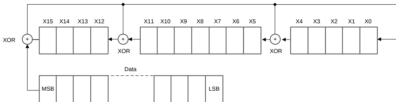
图 21. CCITT-16 CRC Module Block Diagram
