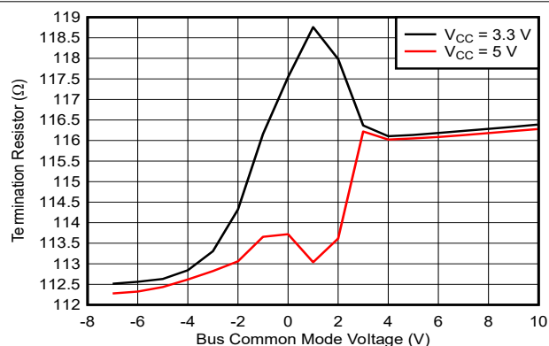
图 5-2. 端接电阻器与总线共模电压之间的关系
