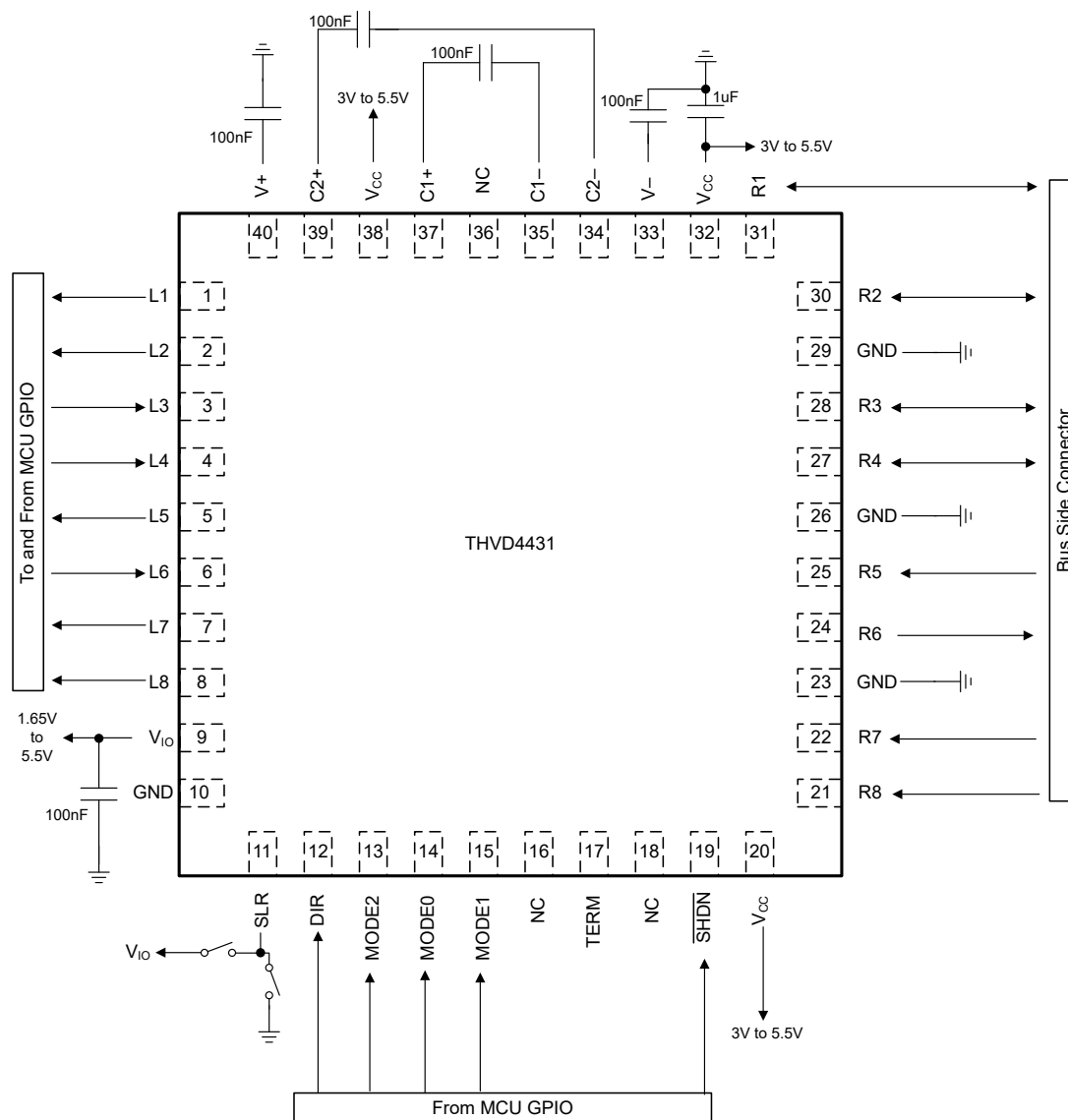
图 8-5. THVD4431 的典型应用图
