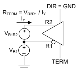
图 6-9. 端接电阻器测量
