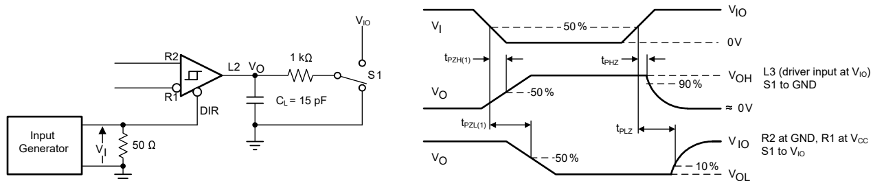
图 6-7. 半双工模式下 RS-485 接收器启用和禁用时间测量
