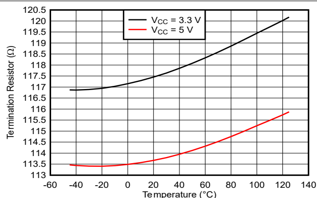
图 5-1. RS-485 端接电阻器与温度之间的关系
