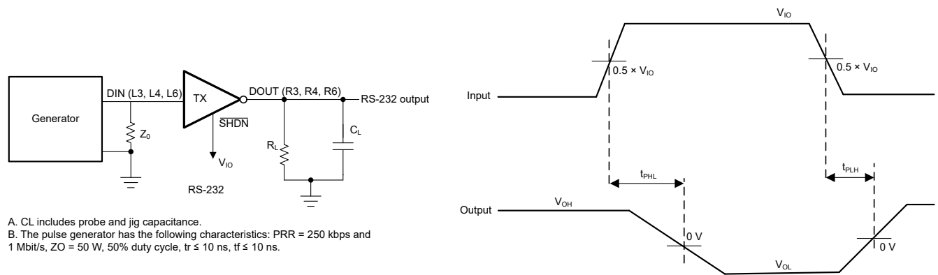
图 6-16. RS-232 驱动器传播延迟，脉冲偏移
