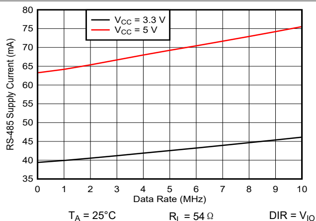
图 5-14. RS-485 20Mbps 电源电流与信号传输速率间的关系
