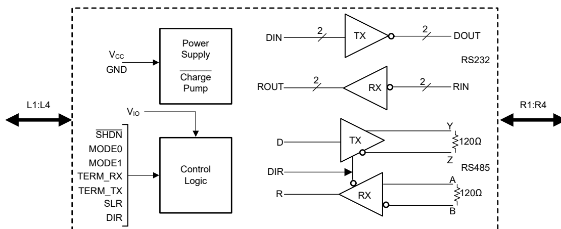
图 7-1. THVD4421 方框图
