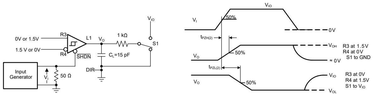
图 6-8. TX 被禁用时 RS-485 接收器从关断开始的启用时间测量全双工模式
