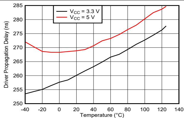
图 5-11. RS-485 500kbps 驱动器传播延迟与温度间的关系
