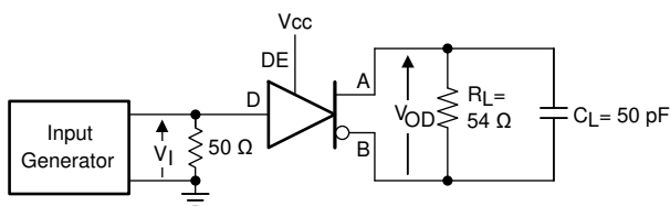
图 6-3. 驱动差分输出上升和下降次数以及传播延迟的测量
