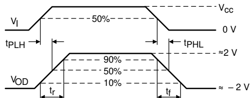
图 6-3. 驱动差分输出上升和下降次数以及传播延迟的测量
