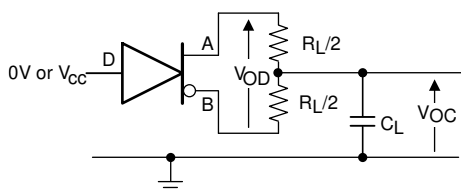
图 6-2. 具有 RS-485 负载的驱动器差分 and 共模输出的测量
