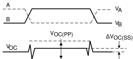
图 6-2. 具有 RS-485 负载的驱动器差分 and 共模输出的测量
