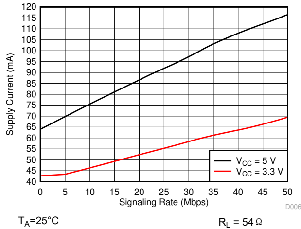
图 6-9. THVD2450 电源电流与信号速率之间的关系
