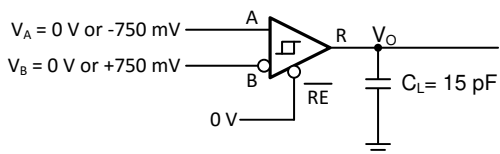
图 6-9. 失效防护延迟测量
