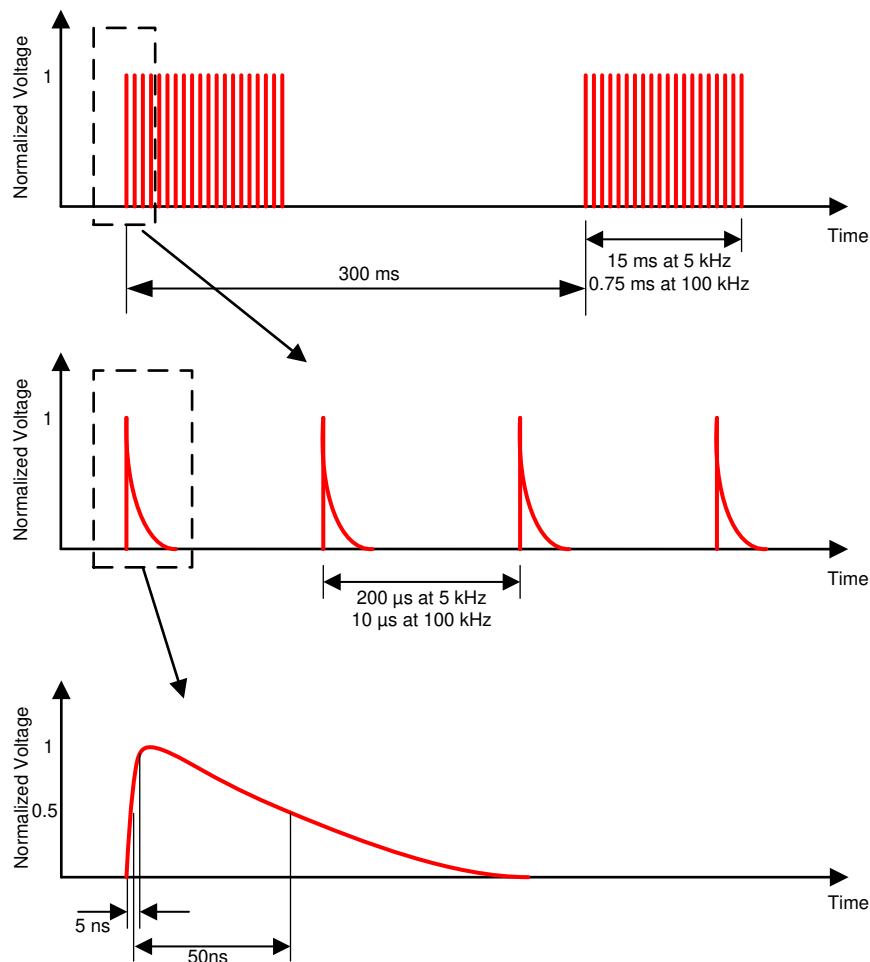
图 8-4. EFT 电压波形
