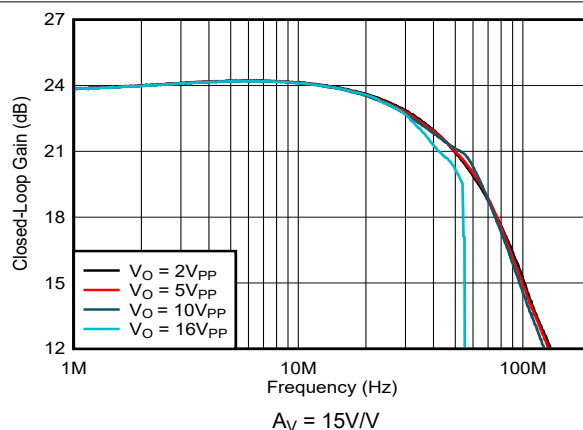
图 5-10. 大信号频率响应与 V_O 间的关系
