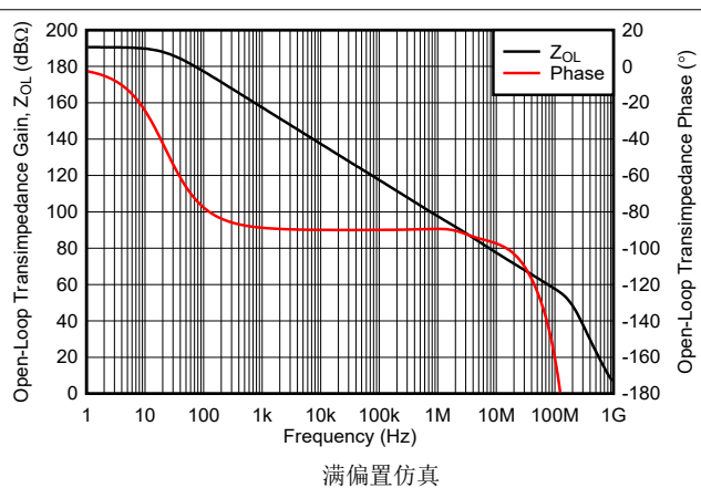
图 5-20. 开环跨阻增益和相位与频率间的关系
