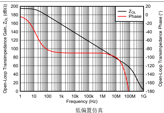
图 5-22. 开环跨阻增益和相位与频率间的关系
