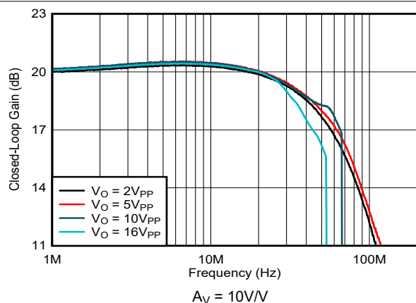
图 5-9. 大信号频率响应与 V_O 间的关系
