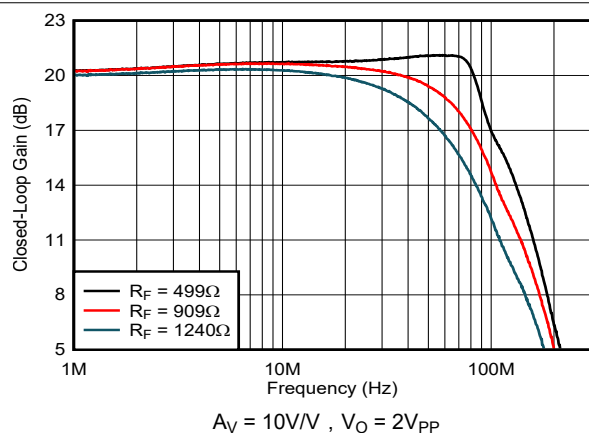
图 5-7. 微小信号频率响应与 R_F 间的关系
