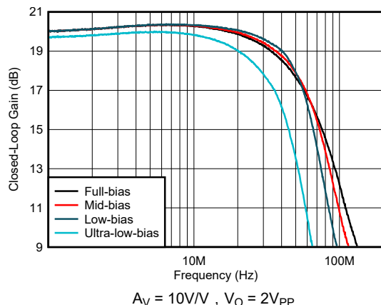
图 5-11. 小信号频率响应与偏置模式间的关系
