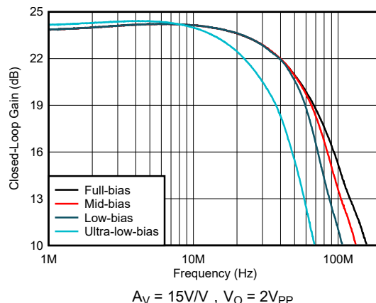
图 5-12. 小信号频率响应与偏置模式间的关系
