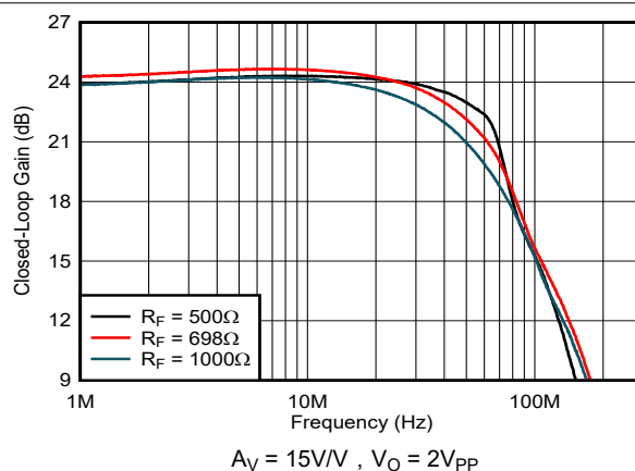
图 5-8. 微小信号频率响应与 R_F 间的关系
