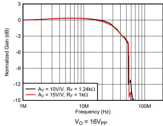
图 5-2. 大信号频率响应
