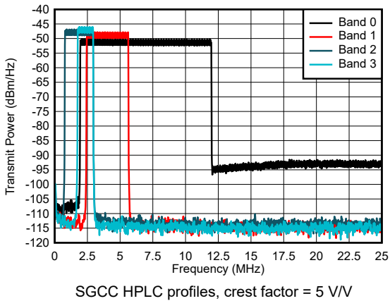
图 5-3. Out-of-Band Suppression
