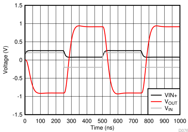
图 10-18. Time-Domain Waveform
