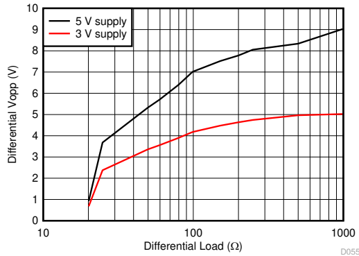
图 6-55. Maximum V_{opp} vs R_{load}
