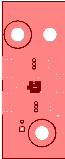
Layer 3 – GND
