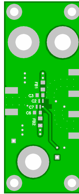
BOTTOM
