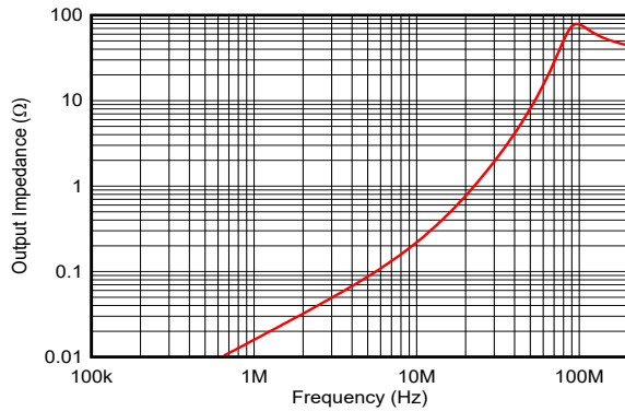
图 5-7. Closed-Loop Output Impedance
