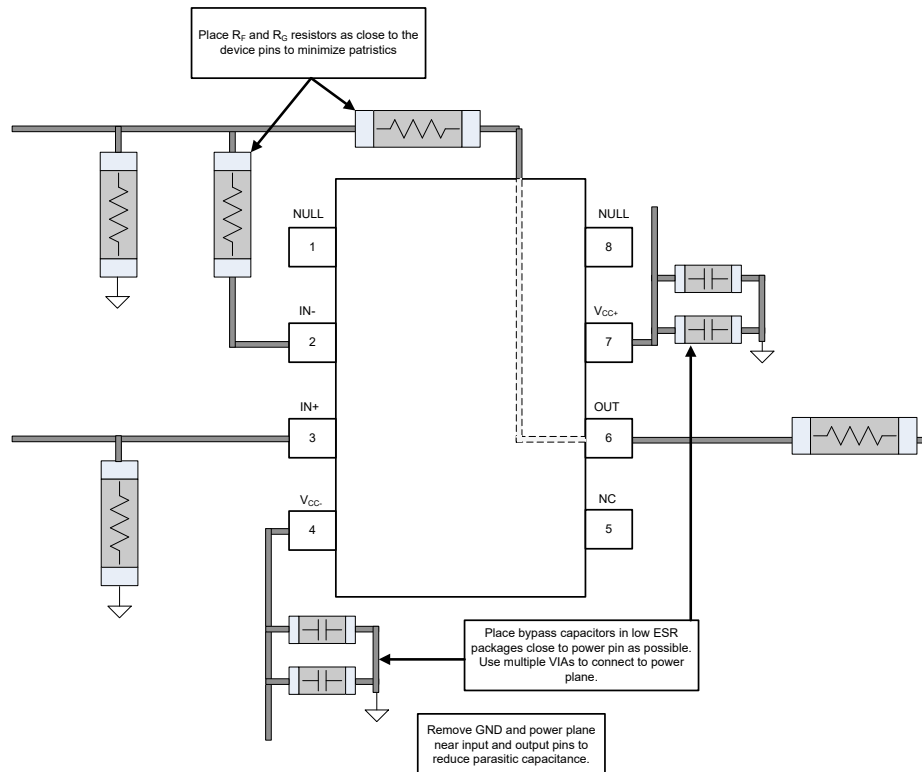
图 7-4. Layout Recommendations
