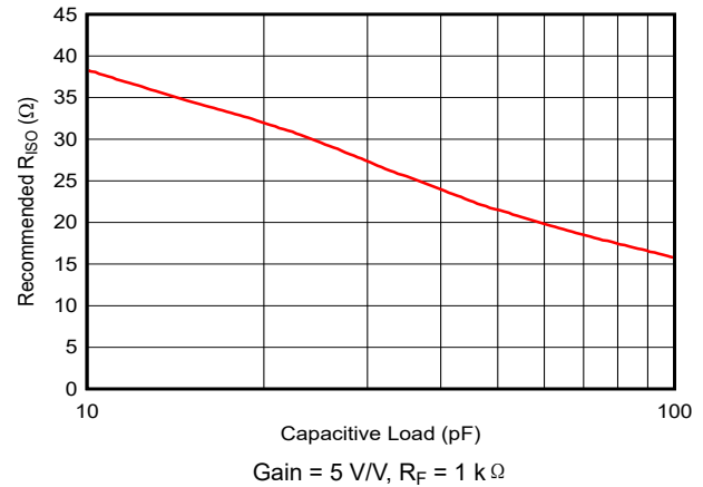
图 7-8. Recommended R_{ISO} vs Capacitive Load
