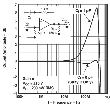
图 7-11. 输出幅度与频率间的关系
