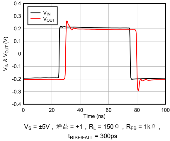
图 5-31. 小信号脉冲响应
