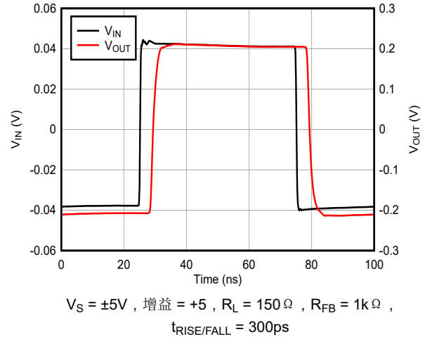
图 5-32. 小信号脉冲响应
