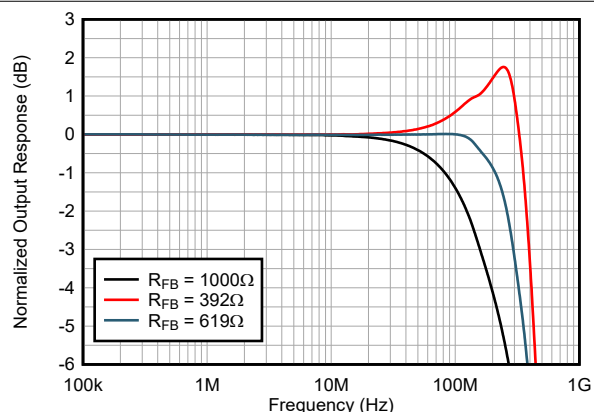
图 5-26. 归一化输出响应与频率间的关系
