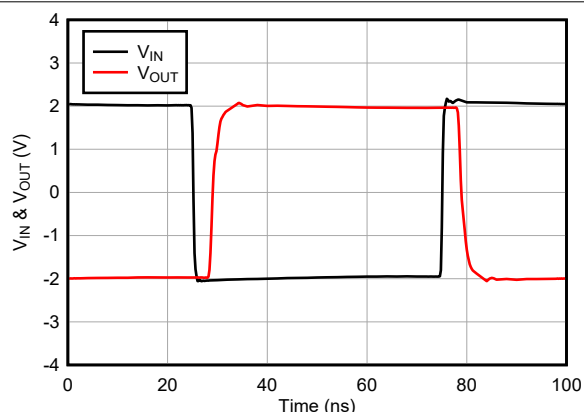
图 5-37. 大信号脉冲响应
