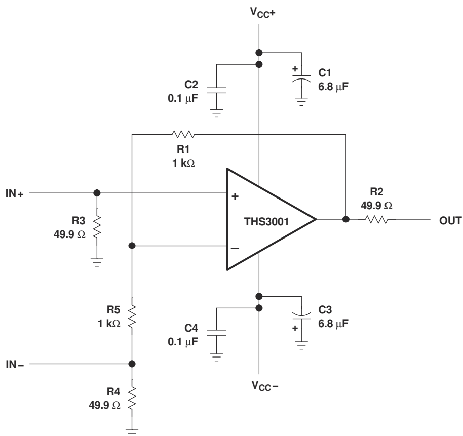
图 8-1. THS3001 评估板原理图
