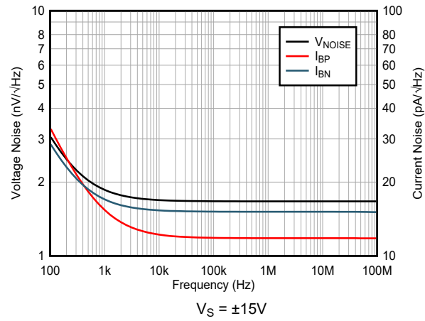
图 5-10. 电压噪声和电流噪声与频率间的关系
