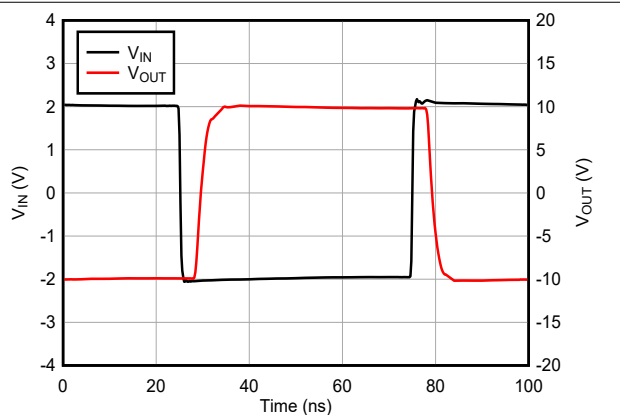
图 5-38. 大信号脉冲响应
