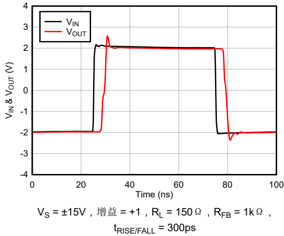
图 5-33. 大信号脉冲响应
