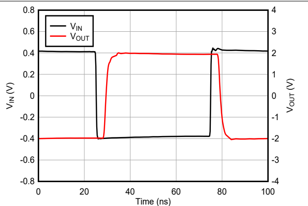
图 5-37. 大信号脉冲响应
