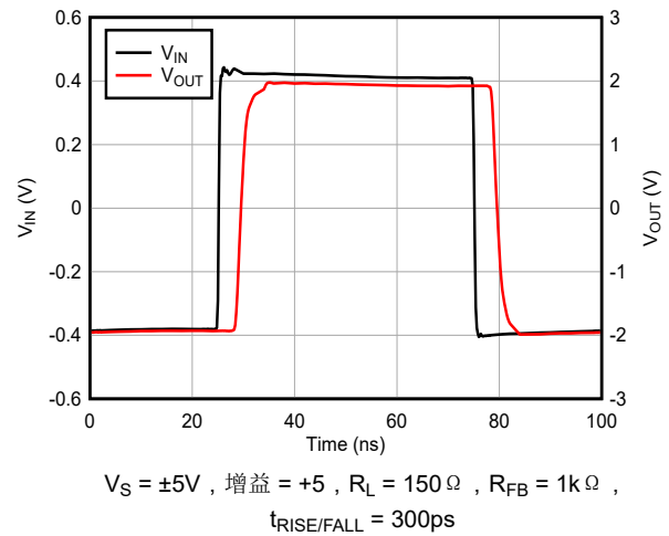
图 5-36. 大信号脉冲响应
