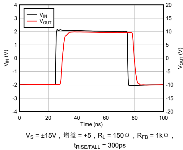
图 5-35. 大信号脉冲响应
