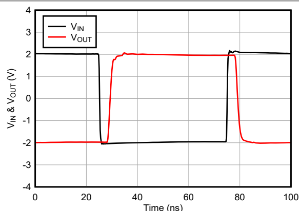
图 5-38. 大信号脉冲响应
