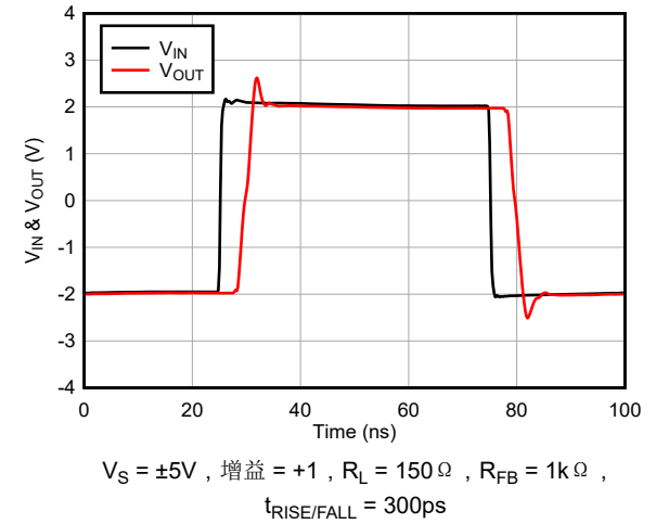
图 5-34. 大信号脉冲响应
