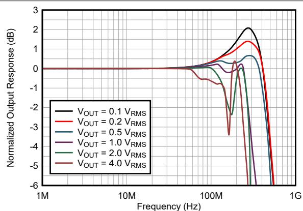
图 5-28. 归一化输出响应与频率间的关系
