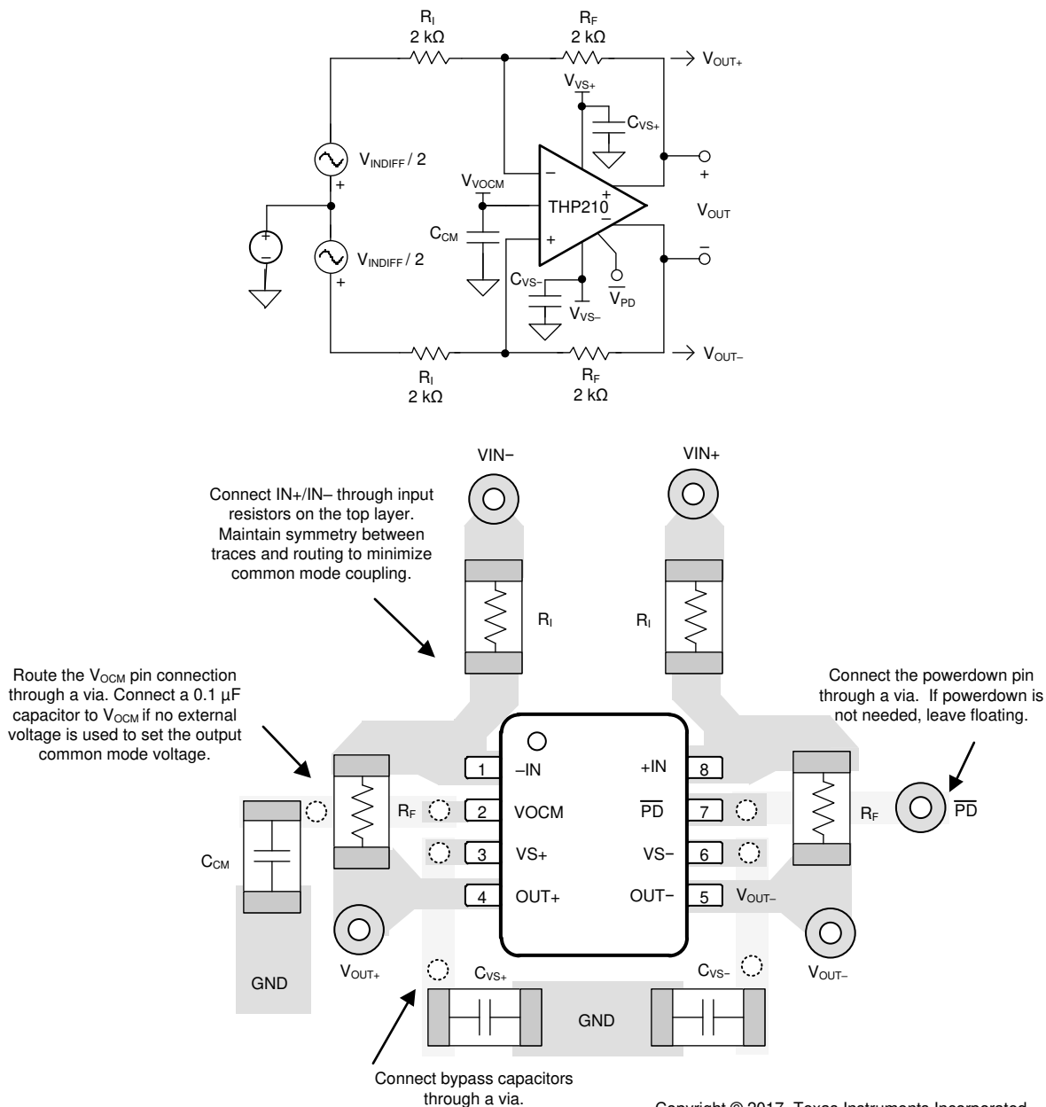
图 11-1. Example Layout
