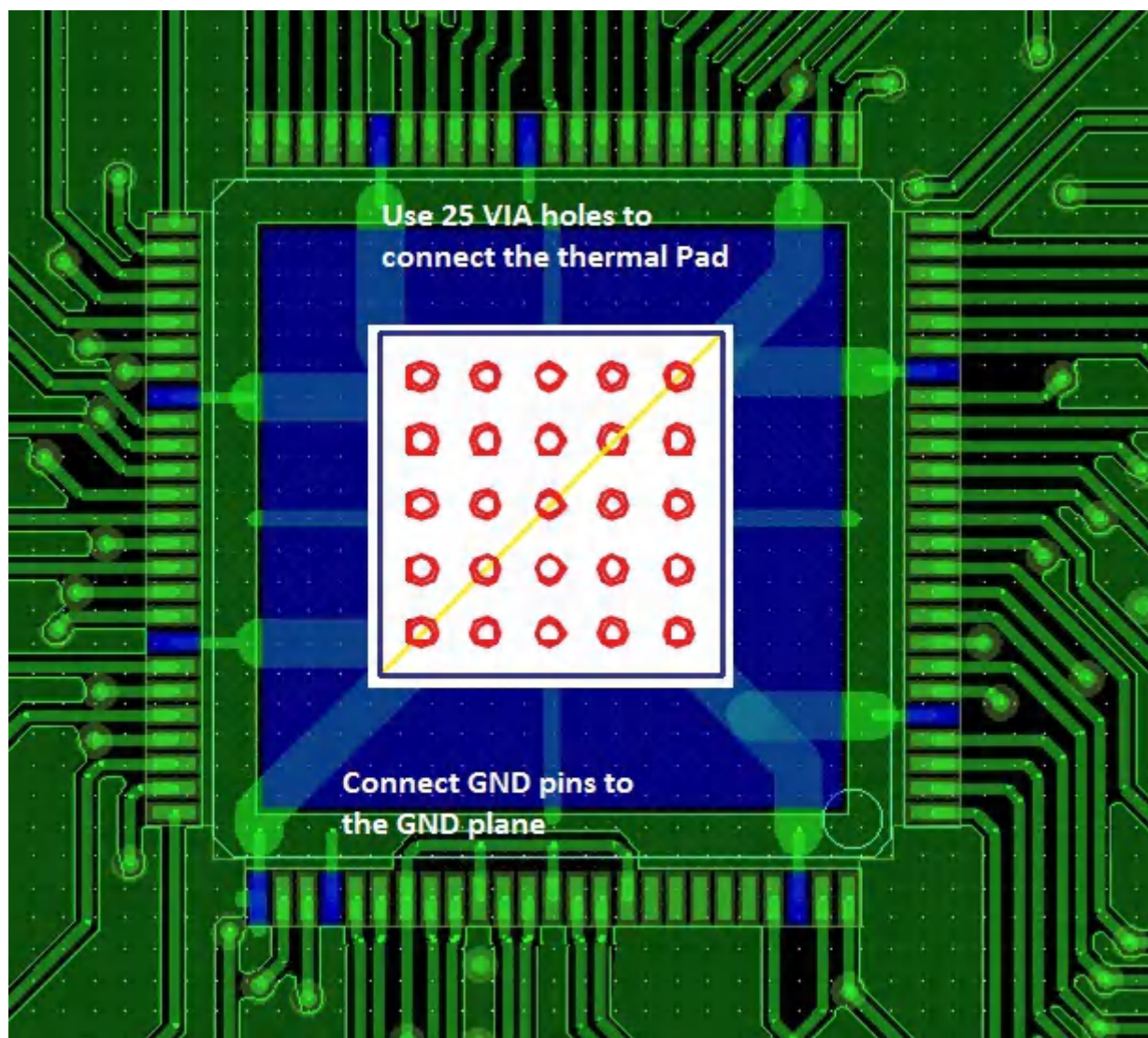
图 7-9. Ground Routing
