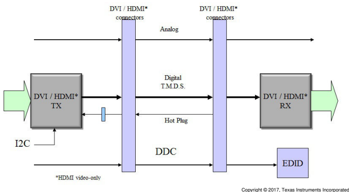
TFP401A-Q1 框图
