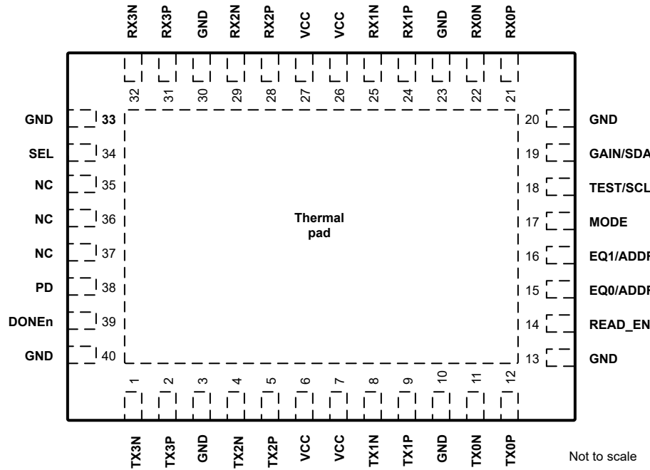
图 4-1. RGF 封装，40 引脚 VQFN (俯视图)
