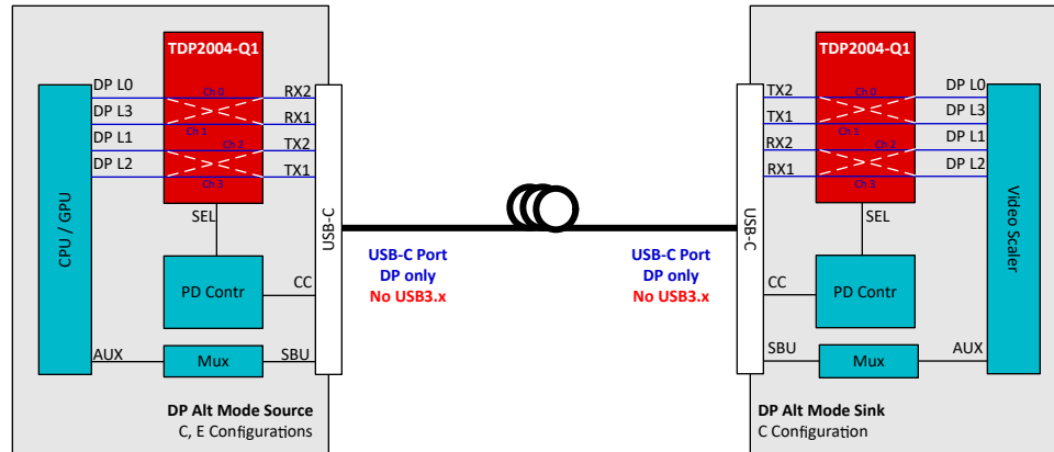
图 7-7. USB-C 应用
