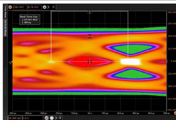
图 7-5. TP3_EQ 处无转接驱动器的 DP 2.1 Tx 符合性眼图
