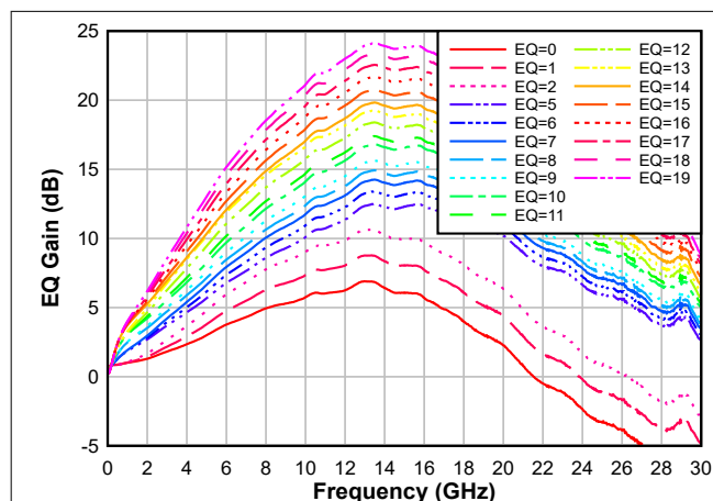
图 5-1. 典型 EQ 增益与频率间的关系
