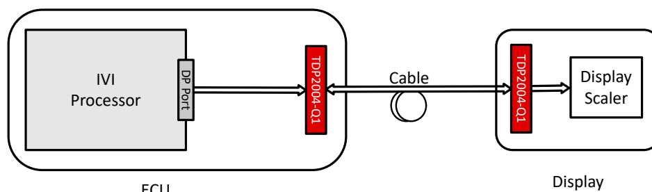
图 7-1. 典型应用
