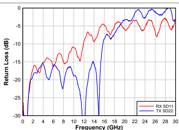
图 5-2. 典型差分回波损耗
