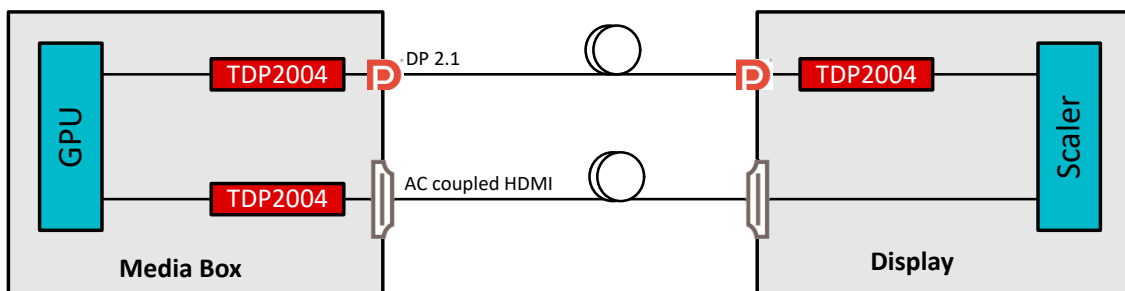
典型应用
