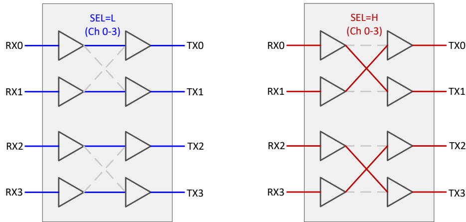
图 6-1. 交叉点多路复用器操作的信号流程图
