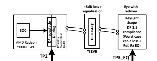
图 7-4. 带转接驱动器的典型 20Gbps (UHBR20) DP 2.1 Tx 兼容性通道设置
