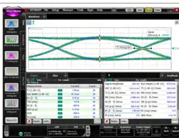
图 5-4. 通过 TDP2004-Q1 (20Gbps 时)
