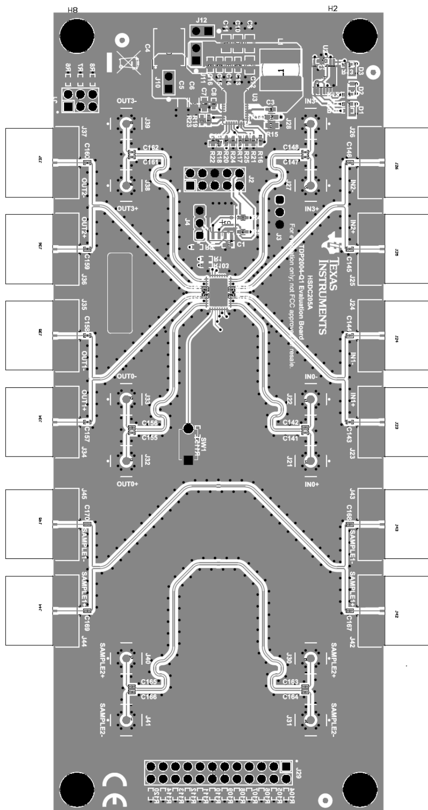
图 7-8. TDP2004-Q1 布局示例 — TI 评估板的子部分
