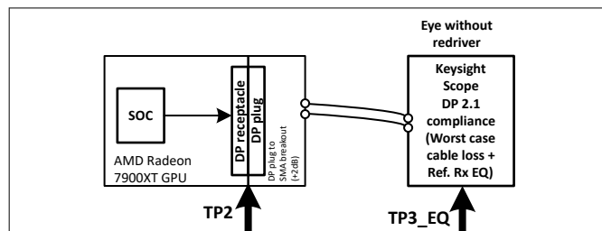
图 7-3. 不带转接驱动器的典型 20Gbps (UHBR20) DP 2.1 Tx 兼容性通道设置
