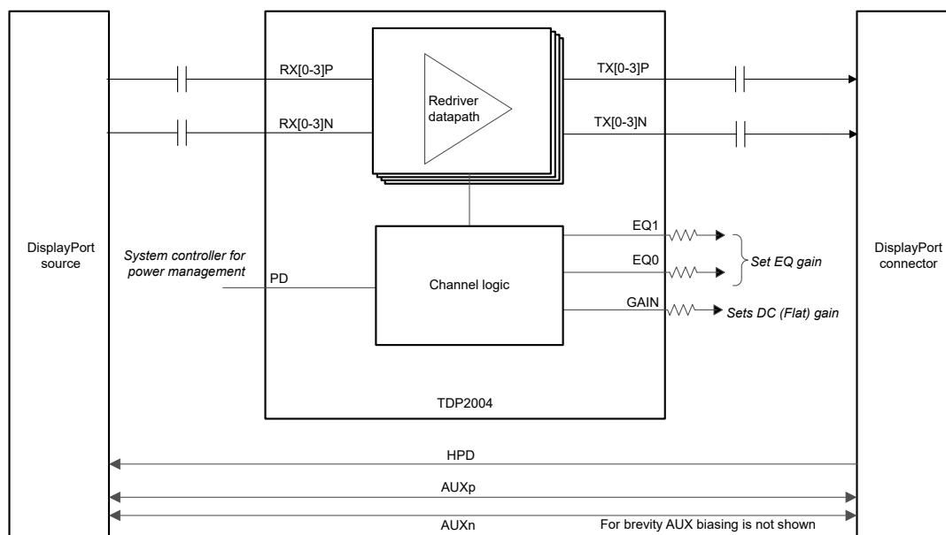
图 7-2. DP 2.1 信号调节的简化版原理图
