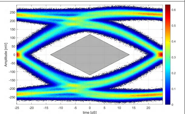
图 7-6. TDP2004 在 TP3_EQ 处用于信号调节的 DP 2.1 Tx 符合性眼图
