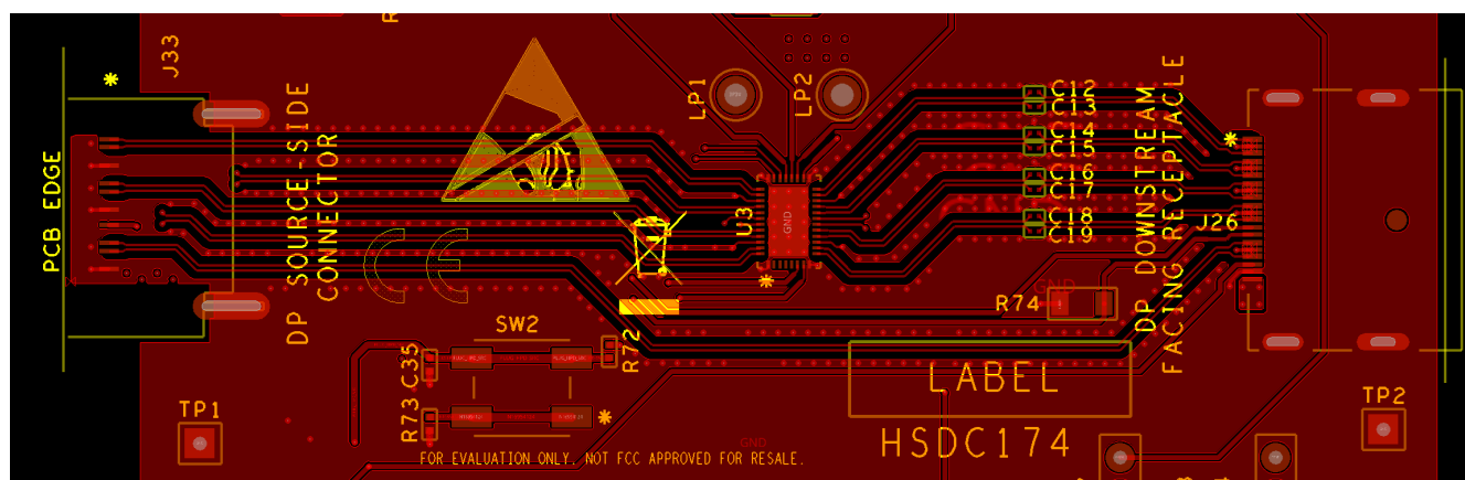
图 7-7. TDP2004 布局示例 - 具有 DP 连接器的 TI 评估板的子部分
