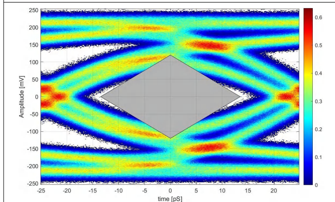
图 7-5. TP3_EQ 处无转接驱动器的 DP 2.1 Tx 符合性眼图
