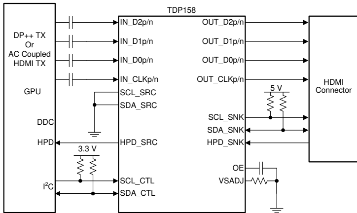
简化原理图
