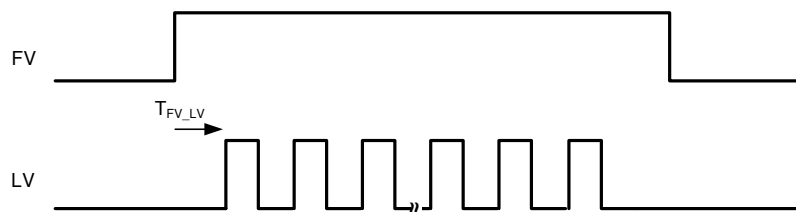
图 7-7. Minimum FV to LV
