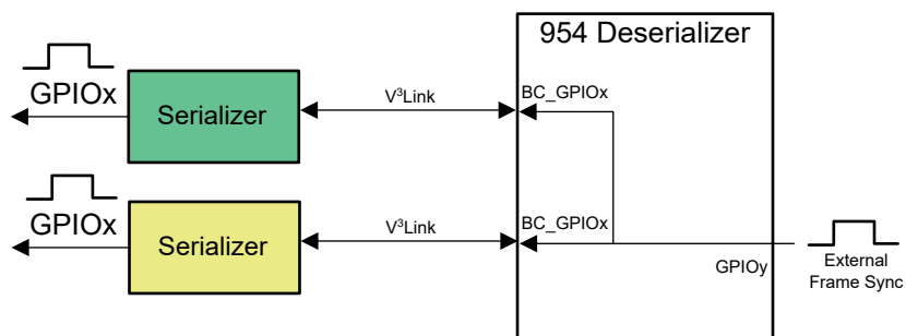
图 7-16. External FrameSync
