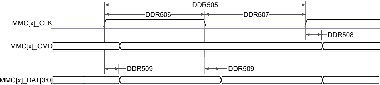
图 6-95. MMC1/2 - UHS-I DDR50 - 发送模式
