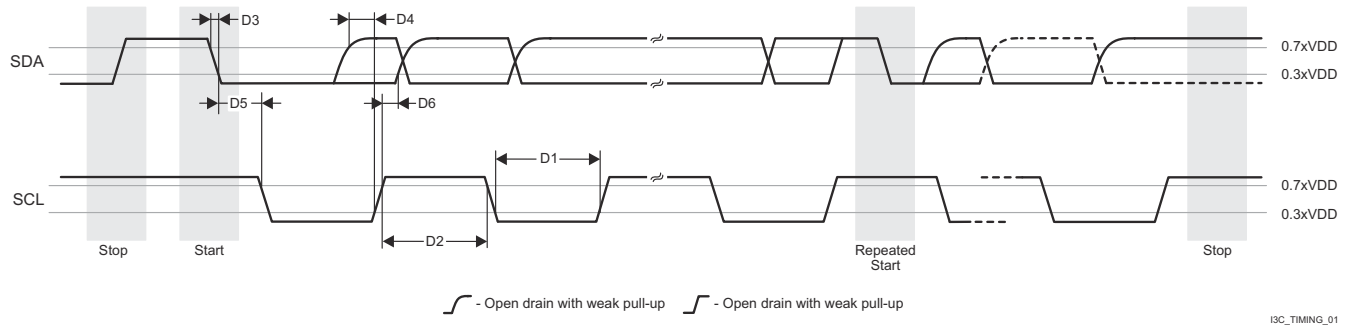
图 6-69. I3C 开漏时序
