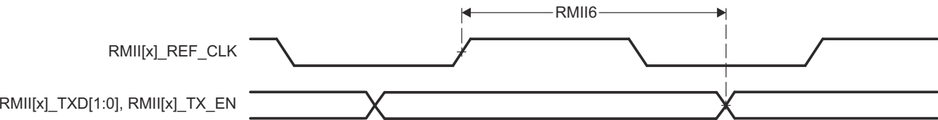
图 6-38. RMII[x]_TXD[1:0] 和 RMII[x]_TX_EN 开关特性 - RMII 模式
