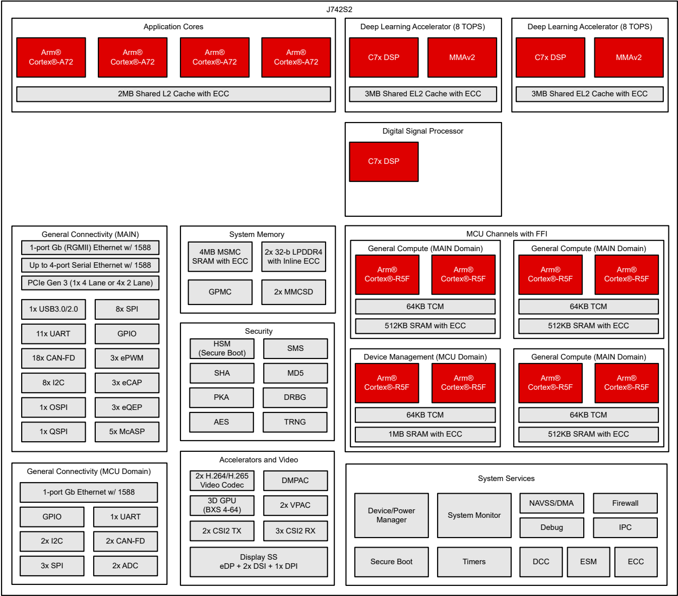
图 3-1. 功能方框图
