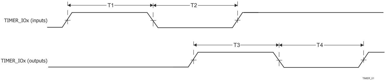
图 6-114. 计时器时序
