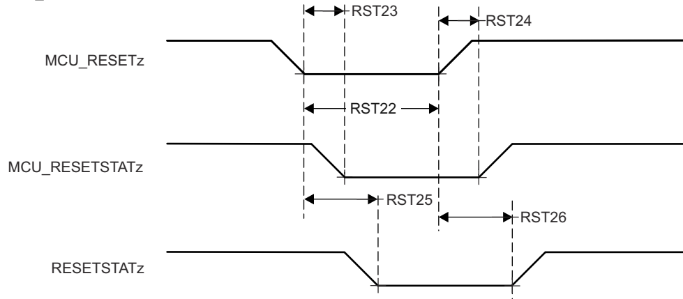
图 6-14. MCU_RESETz 启动 ; MCU_RESETSTATz 和 RESETSTATz 时序要求和开关特性
