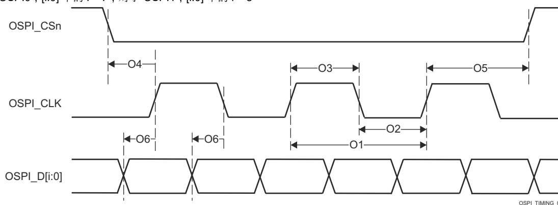
图 6-106. OSPI 开关特性 - DDR
