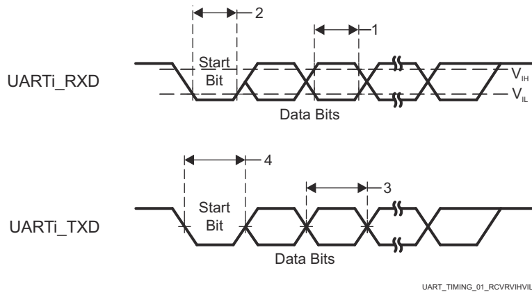
图 6-115. UART 时序
