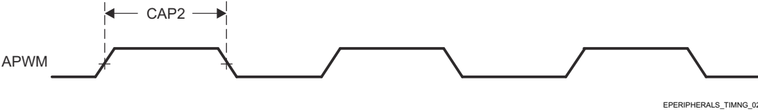
图 6-45. eCAP 输出时序
