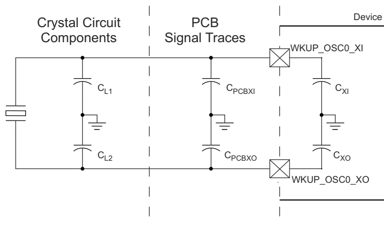
图 6-25. Load Capacitance
