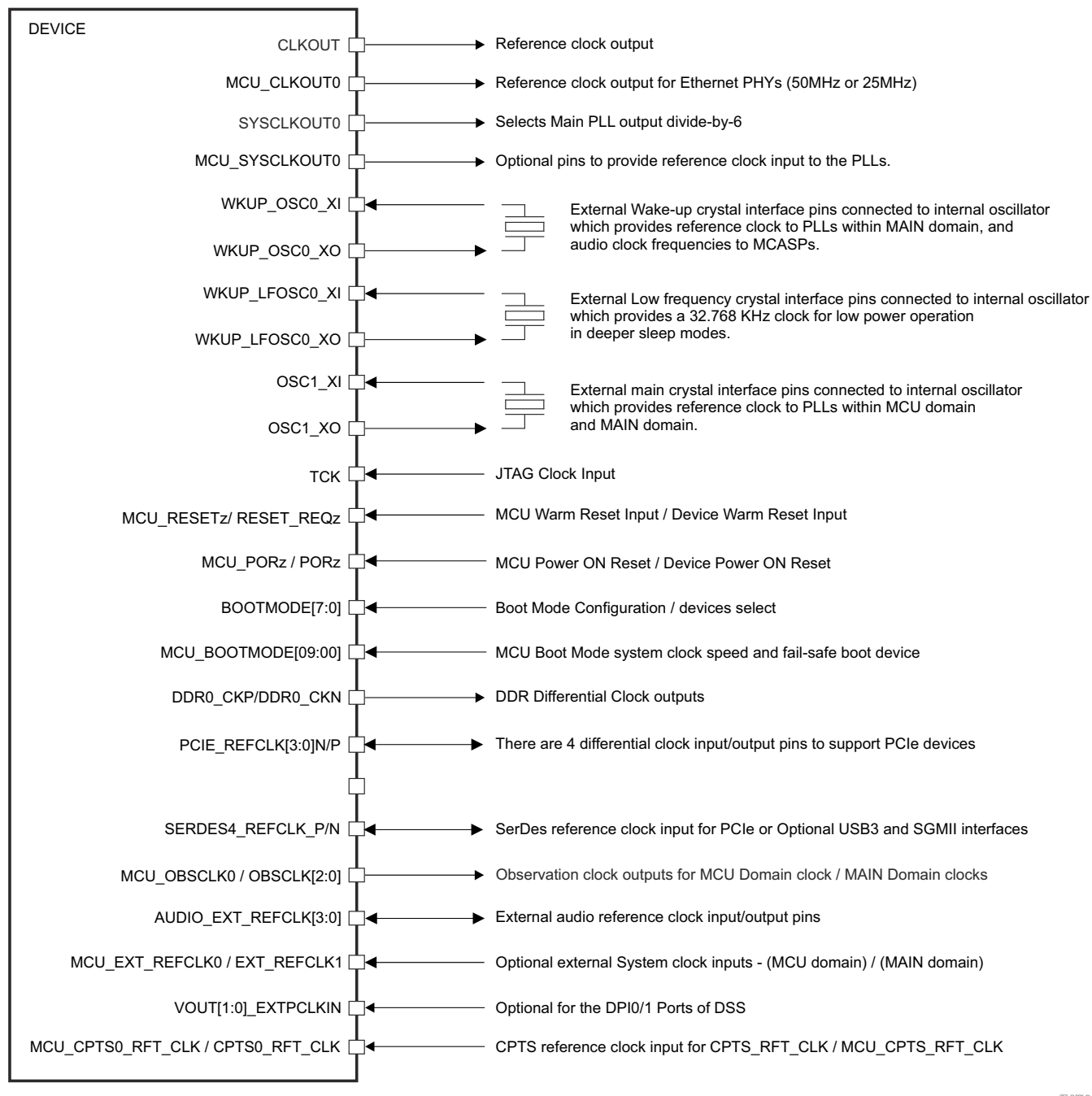
图 6-22. Input Clocks Interface
