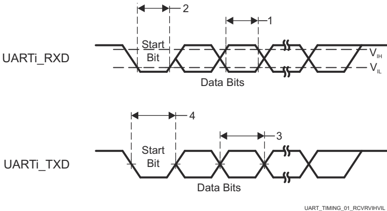
图 6-112. UART 时序
