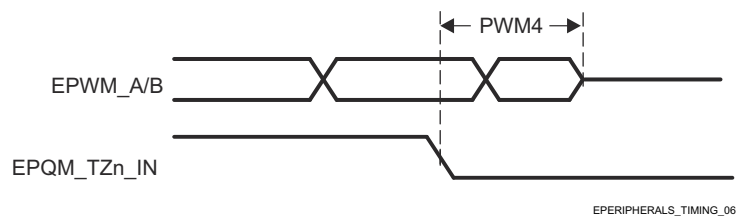
图 6-49. EPWM_A/B 和 ePWM_TZn_IN 高阻态输入时序
