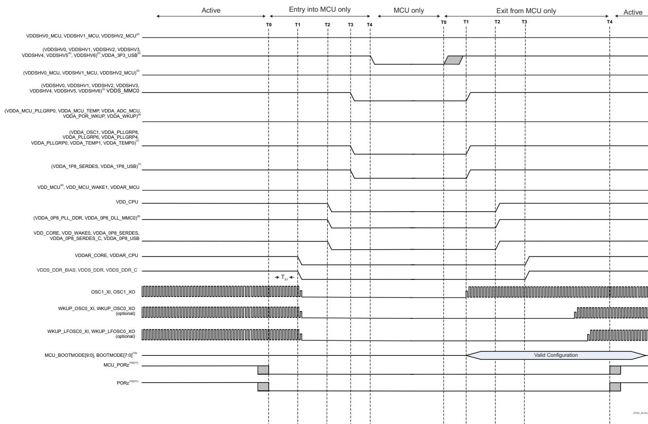
图 6-7. 独立的 MCU 域和 Main 域,仅 MCU 时序的进入和退出
