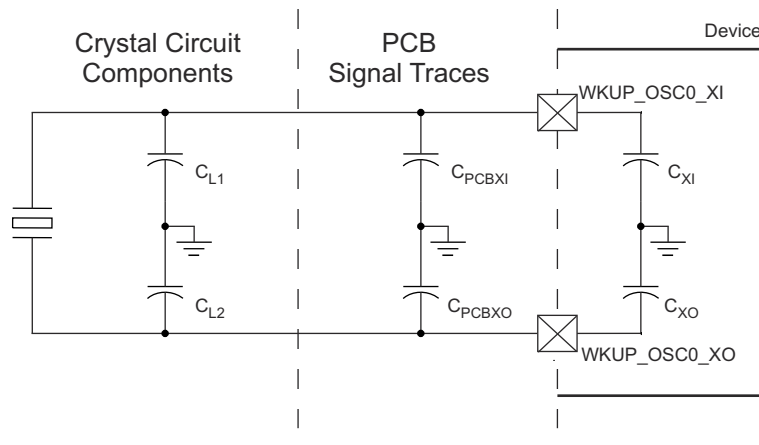
图 6-25. 负载电容
