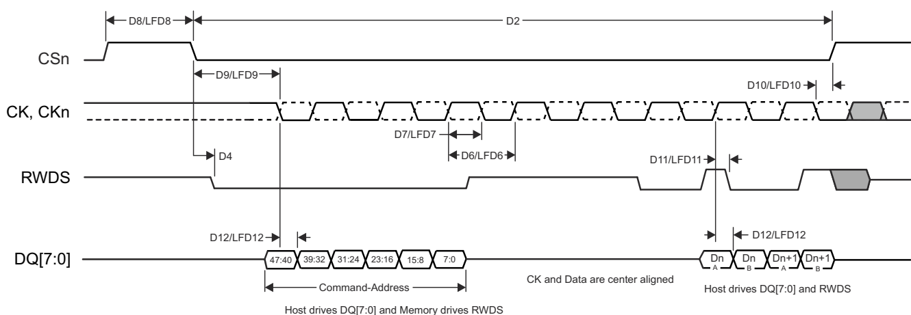
图 6-66. HyperBus 时序图 - 发送器模式
