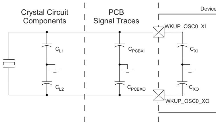
图 6-25. 负载电容
