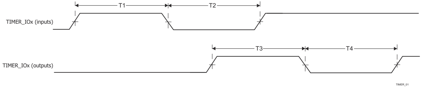
图 6-111. 计时器时序
