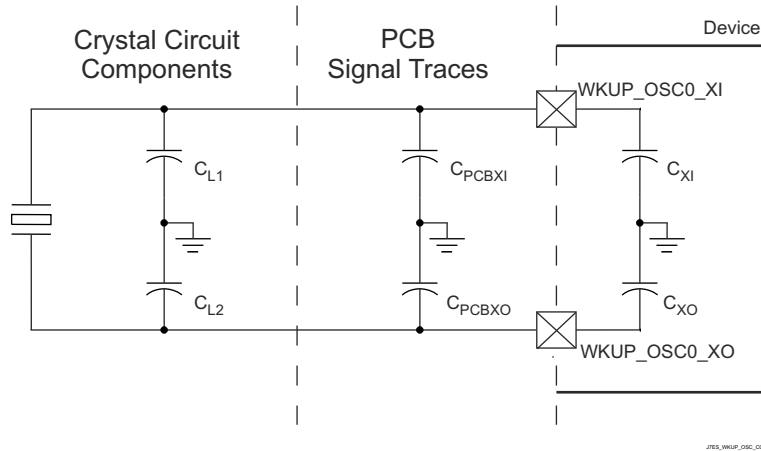
图 7-25. Load Capacitance
