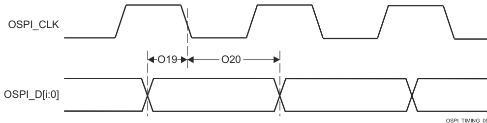
图 6-99. OSPI0 时序要求 - 具有内部 PHY 环回的 PHY SDR
