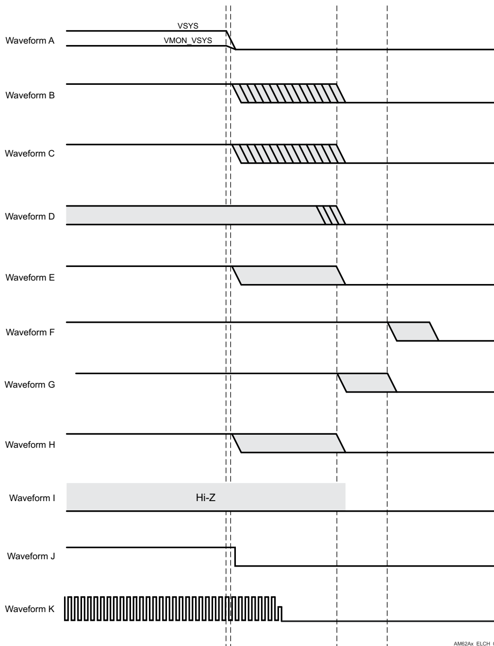
图 6-6. 下电时序
